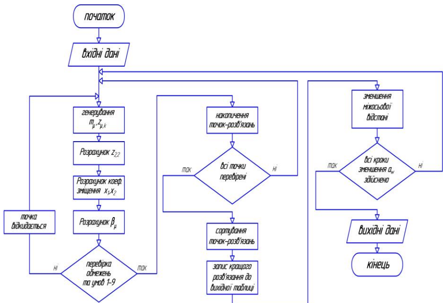
Рисунок 2 – Схема алгоритму проектування
