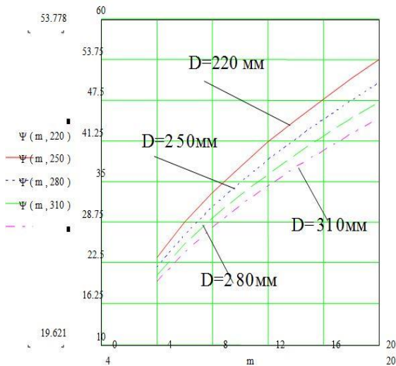
Рис. 2 – Изменение угла контакта зуба фрезы с обрабатываемой рейкой
