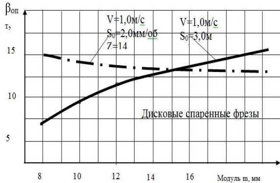
Рис.1 – Зависимость изменения оптимального угла рассогласования \beta_{опт} от обрабатываемого модуля зубчатой рейки при различных технологических режимах обработки
