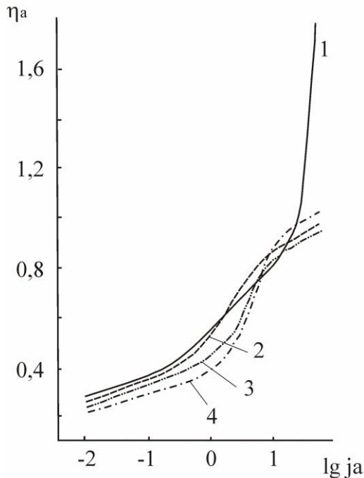
Рис. 2 – Поляризаційні залежності виділення кисню в розчинах КОН різної концентрації (моль·дм -3 ): 1 – 1,0; 2 – 10, 3 – 5,0; 4 – 7,0.
