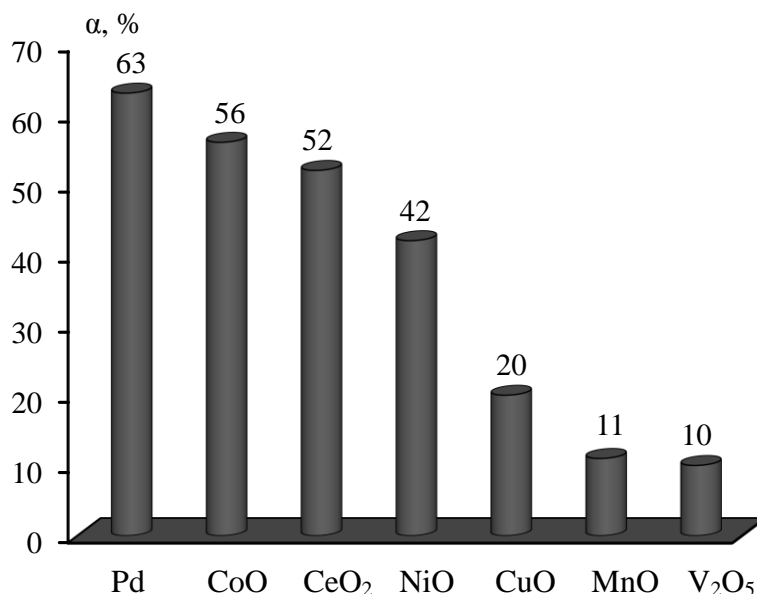
Рис. 3 – Порівняльна діаграма каталізаторів за ступенем конверсії для реакції безплатицевого окиснення бензолу
