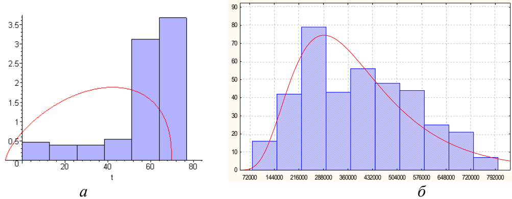
Рисунок 5 – Гістограми і теоретичесие кривые распределения нарушений работоспособности автономного отопителя: a - гарантийный пробег; б - послегарантийный пробег
