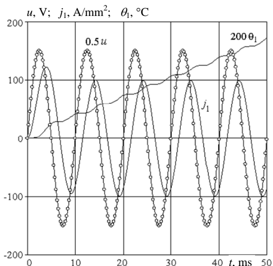
Рис. 1. Электрические и тепловые характеристики ЛЭМП при отсутствии обмотки якоря
