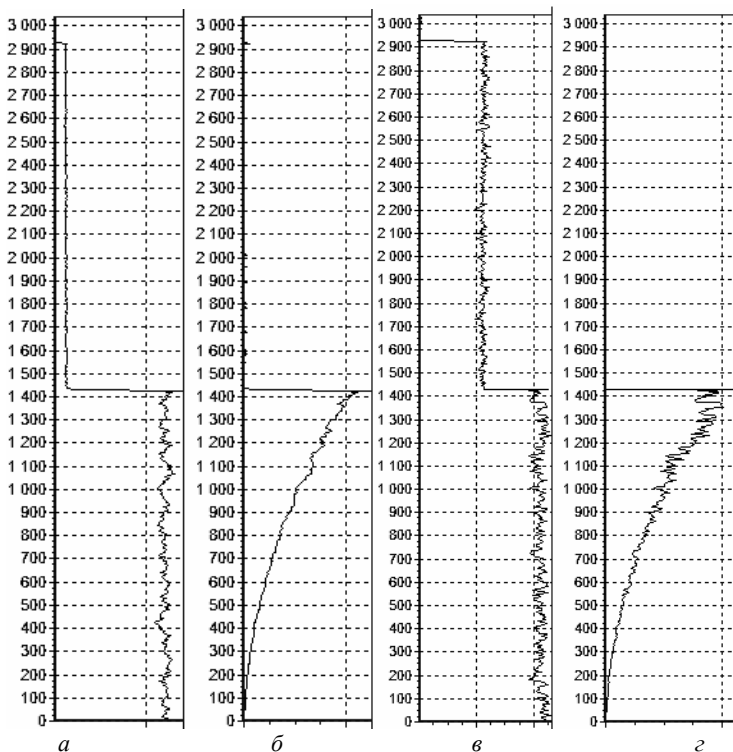
Рис. 5 – Мощность сигнала ( a и в ) и сечение рассеяния ( б и г ) для q=10 ( a и б ) и q=10 ( в и г ), усреднённые по 1464 радиолокационным развѳрткам
