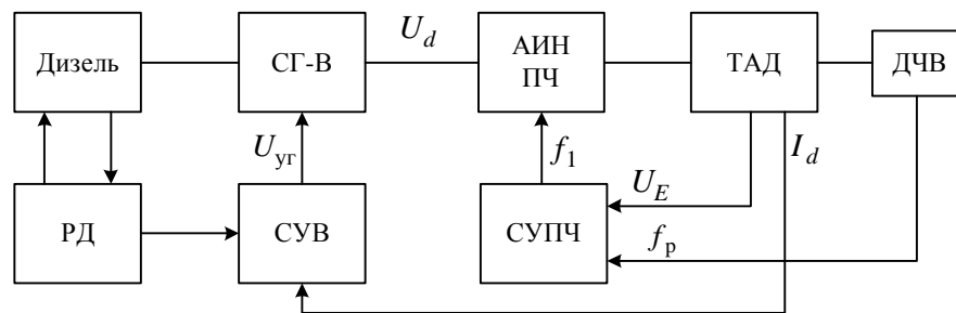
Рисунок 1 – Структурная схема САР электропередачи дизель-поезда
