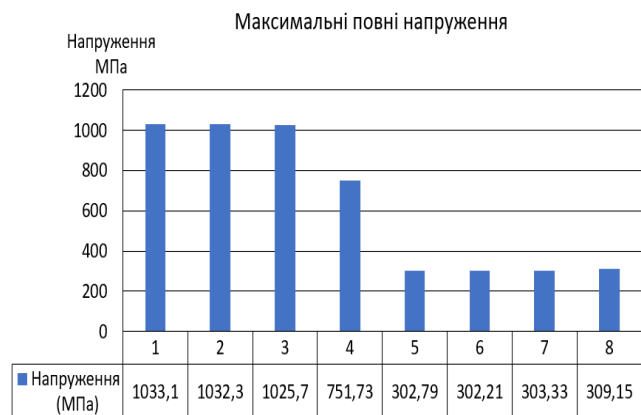
Рисунок 7 – Максимальні еквівалентні напруження (див. табл. 1)
