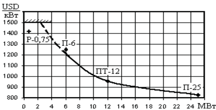
Рис. 2. Удельные инвестиции на реализацию проекта по установке малых паровых конденсационных турбин в ценах на начало 2011 г.
