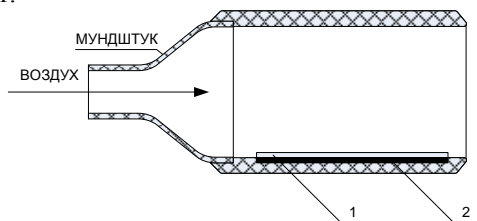
Рис. 5. Термокондуктометрический датчик
