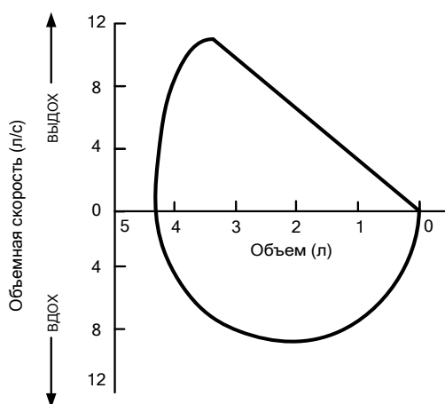
Рис. 1. Петля «поток-объем»
