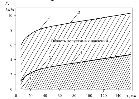
Рис. Результаты расчета величины напряжений, возникающих вследствие гидростатического давления и области допустимых значений давления при затвердевании в кокиле фасонной отливки из сплава АК5М
