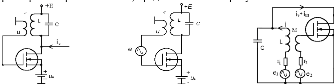
Рис.1. Схемы автогенераторов
