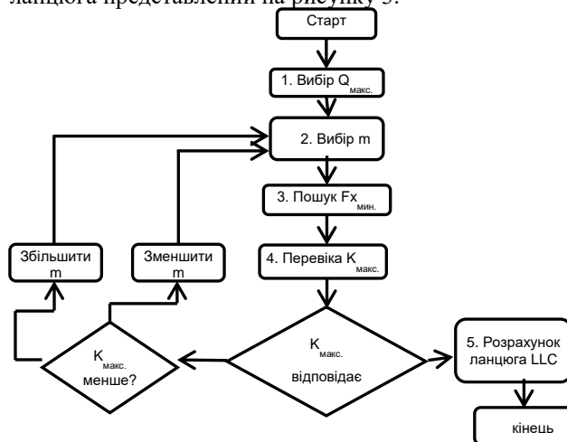
Рис. 3. Алгоритм розрахунку параметрів резонансного ланцюга
