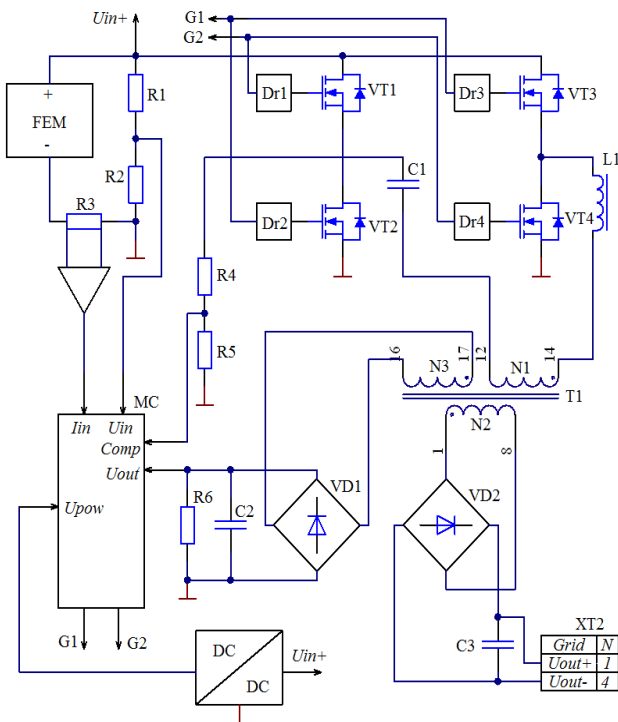
Рис. 8. Функціональна електрична схема DC-DC перетворювача
