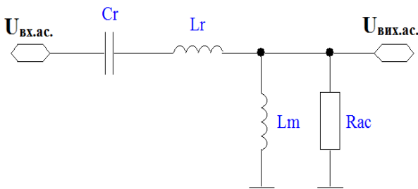
Рис. 2. Еквівалентна схема заміщення резонансної ланцюга LLC
