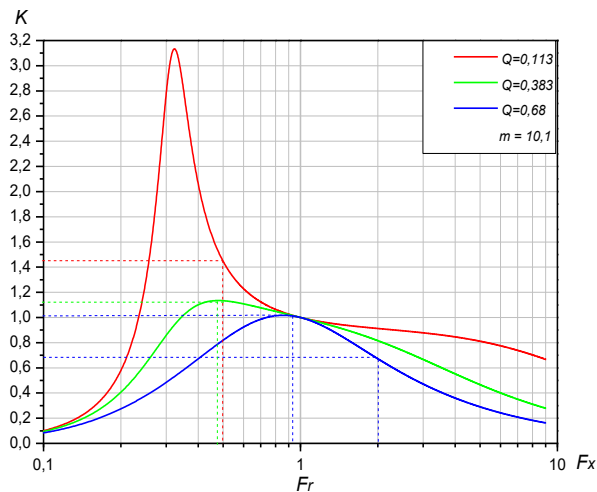
Рис. 6. Залежність коефіцієнта передачі LLC контуру від нормалізованої частоти при заданих значеннях добротності
