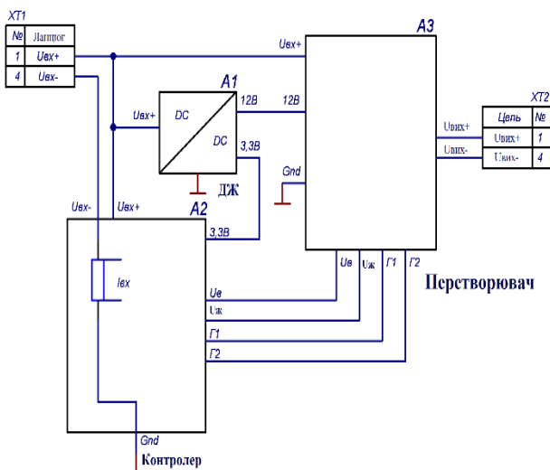
Рис. 9. Принципова електрична схема DC-DC перетворювача
