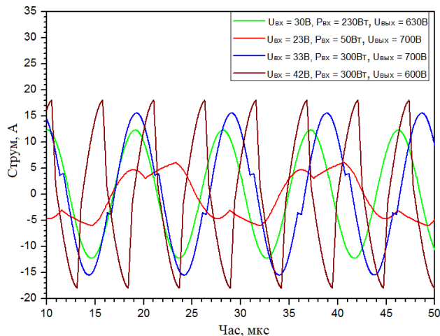
Рис. 7. Модельна тимчасова діаграма струму дроселя
