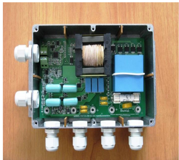
Рис. 10. Розроблений і виготовлений DC-DC перетворювач
