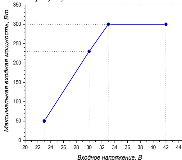
Рис. 5. Залежність максимальної вихідної потужності DC-DC перетворювача від вхідної напруги
