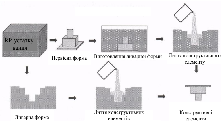
Рисунок 11 - Ланцюг процесів у прямому та непрямому Rapid Tooling
