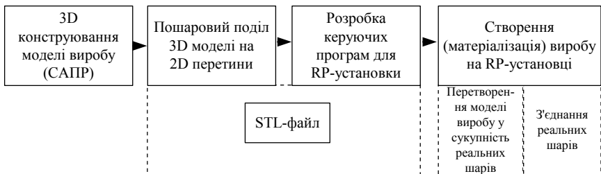
Рисунок 3 – Функціональна схема технологій прискореного формоутворення
