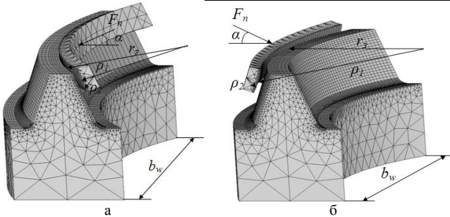
Рисунок 2 – Модели нагружения индентором арочного зуба рейки: а – с вогнутой стороны зуба; б – с выпуклой стороны зуба
