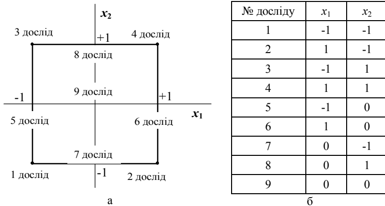
Рисунок. План експерименту: а – графічна інтерпретація, б – таблиця кодованих чинників.
