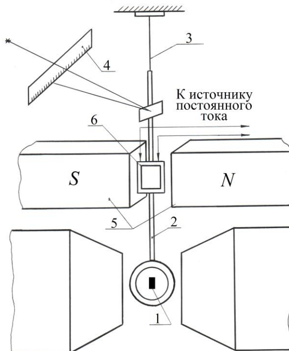
Рисунок 1 – Схема установки для измерения намагниченности насыщения и константы перпендикулярной анизотропии
