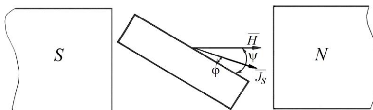
Рисунок 2 - Взаимное расположение векторов напряженности поля и намагниченности
