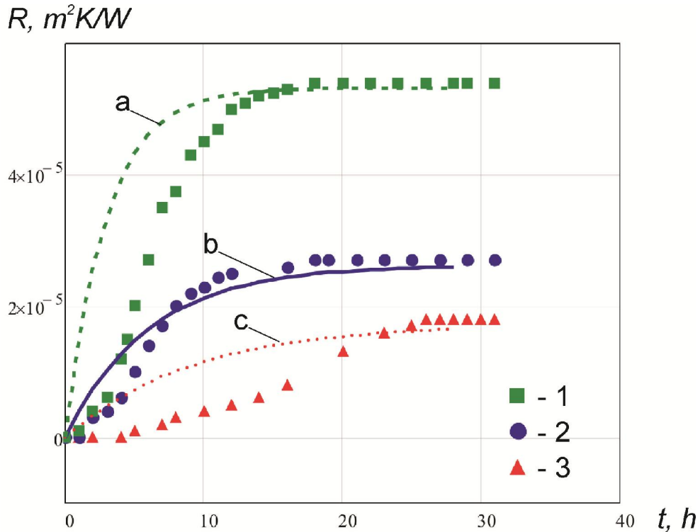
Рис. 6. Термическое сопротивление отложений при накипеобразовании карбоната кальция в круглом канале [10], w=1.2 м/с: 1 и линия а – T_s=64^\circ\text{C} ; 2 и линия б – T_s=51^\circ\text{C} ; 3 и линия с – T_s=44^\circ\text{C}
