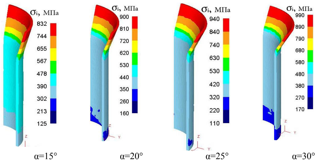
Рис. 8 – Розподіл інтенсивності напружень \sigma_i по об'єму zdeформованої заготовки
