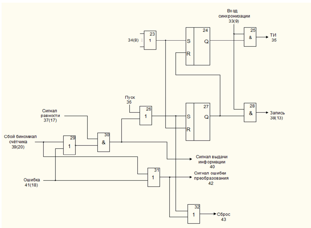
Рис. 3 – Схема устройства управления
