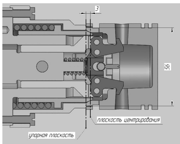
Рис. 3. Предлагаемая схема закрепления
