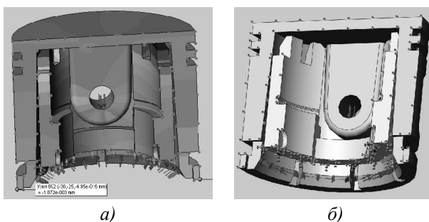
Рис. 1 – Предварительный расчет закрепления а) перемещение (деформация) в наименее жестком месте поршня; б) схема закрепления
