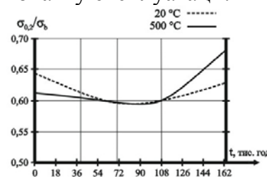
Рис. 2 – Характеристика зміни комплексного показника \sigma_{0,2}/\sigma_b
