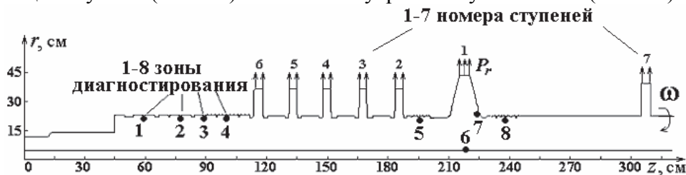
Рис. 1 – Розрахункова схема РВД
