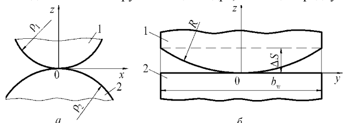
Рисунок 1 – Расчетные модели контакта цилиндров 1 и 2 в плоскости zOx (а) и цилиндра с плоскостью 2 в плоскости zOy (б) в соответствии с решениями новой теории контактной прочности имеют вид [8]:
