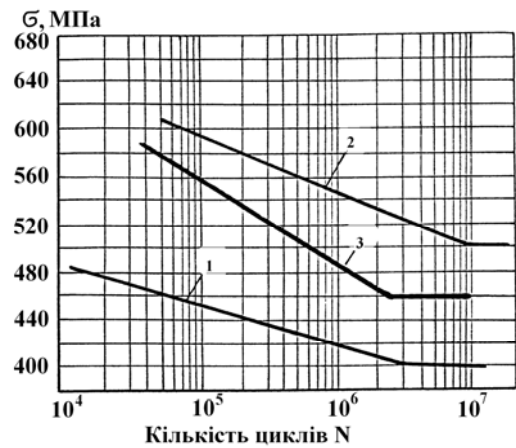
Рис. 6. Графіки Велера для сталі 45 (1) з аморфними детонаційними (2) та плазморовими (3) покриттями із сплаву Fe-B-C [6]
