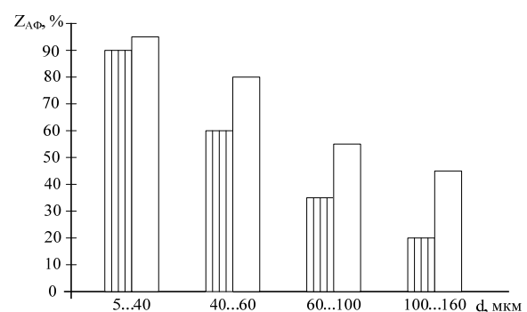
Рис. 1. Вплив розміру частинок порошку із сплаву Fe-B-Si-C на об'ємний зміст аморфної фази при детонаційному напиленні сумішами: - ацетилен-кисень □ ; - пропан-бутан-кисень □.
