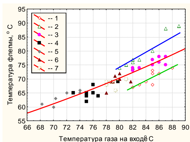
Рис. 2. Зависимость температуры флегмы от температуры газа на входе в аппарат: 1 – КДС-ТБ; 2 – КДС-ТК; 3 – КДС-ТТ; 4 – ХГДС-1; 5 – ХГДС-2; 6 – ХГДС-3; 7 – ХГДС-4.
