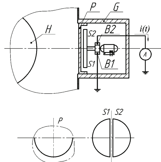
Рисунок 2 – Роторный вольтметр [2]
