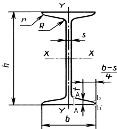
Рис. 3. Схема балки
