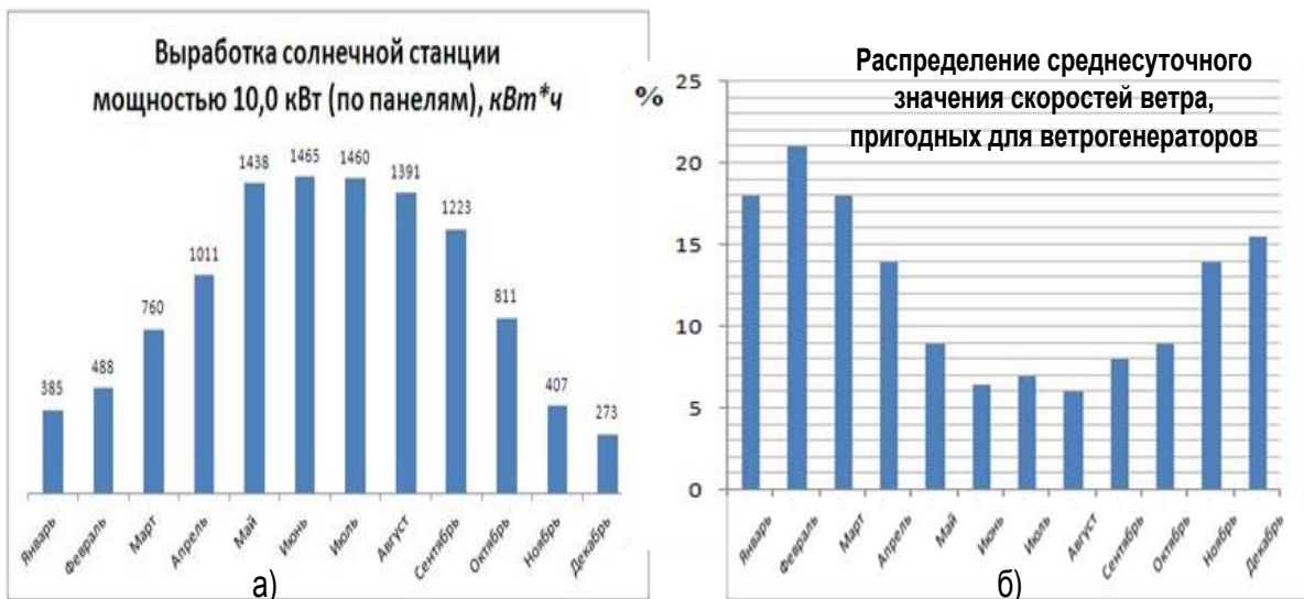
Рисунок 1 – Графики распределения потенциала энергоустановок а) – для солнечных батарей, б) – для ветрогенераторов).
