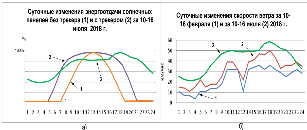
Рисунок 2 – Графики суточного распределения потенциала энергоустановок
