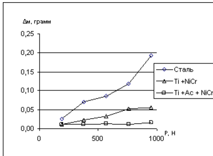
Рис. 3 – Весовой износ образцов при скорости трения 0,5 м/с.
