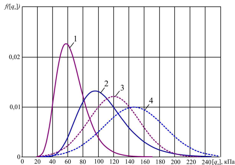
Рис. 2 – Щільності ймовірності розподілу нормативної величини допустимого тиску на ґрунт: 1 – передпосівний обробіток (пухкий ґрунт); 2 – передпосівний обробіток (помірно ущільнений ґрунт); 3 – основний обробіток (ущільнений ґрунт); 4 – основний обробіток (рівноважний ґрунт).
