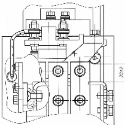
Рис. 3. Узел форсировки привода контактора МК 1221А
