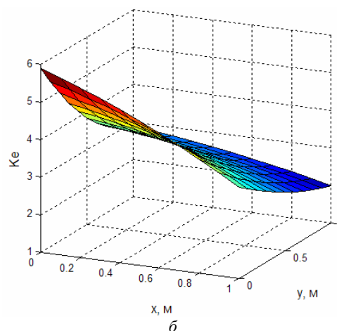
Рис. 5. Поверхности распределения: а) индукций исходного магнитного поля линии электропередачи и магнитного поля с включенной системой; б) уровня компенсации индукции магнитного поля с помощью системы
