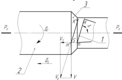
Рисунок 1 – Схема перемещения точек режущей кромки по поверхности резания, во время рабочего цикла: 1-режуща кромка; 2-заготовка; 3 – поверхность резания
