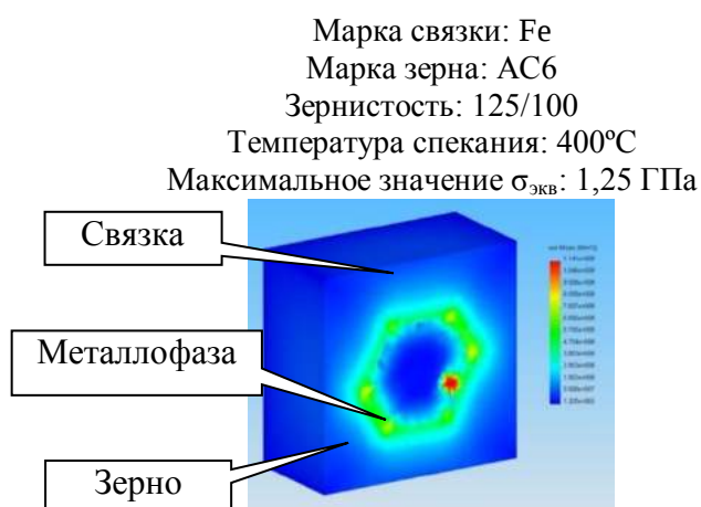
Рис. 1 – Визуализация результатов расчета зависимости эквивалентных напряжений от температуры спекания кругов на металлических связках
