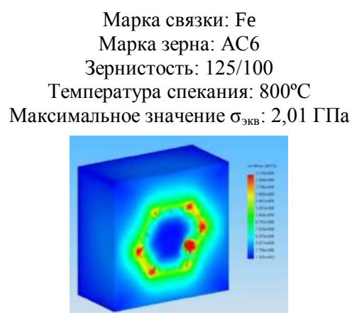
Рис. 1 – Визуализация результатов расчета зависимости эквивалентных напряжений от температуры спекания кругов на металлических связках
