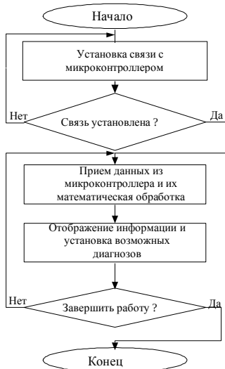
Рис. 5. Алгоритм работы виртуальной части кардиографа
