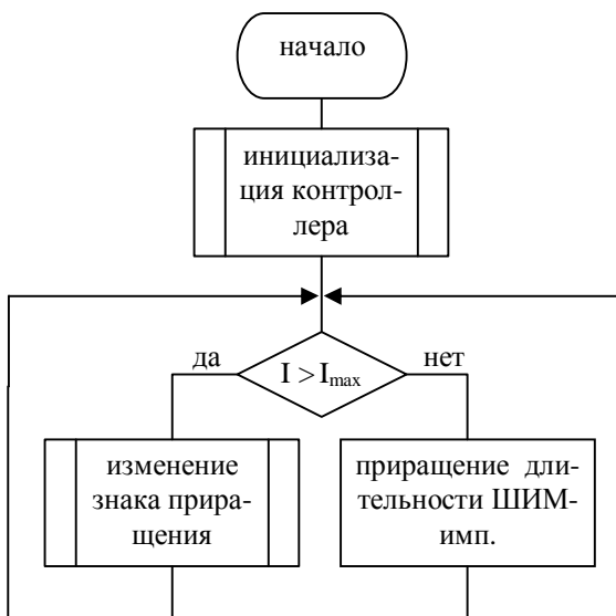
Рис. 3 – Общий алгоритм работы контроллера
