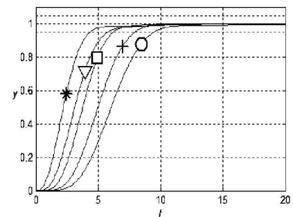
Рис. 5 – Переходные процессы
