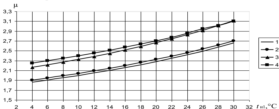
Рис. 1 – Зависимость коэффициента преобразования теплоты \mu от температуры грунтовой воды на входе в испаритель ТНУ t_{н1} .
