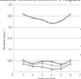
Рисунок 6 – Весовой износ наплавленных образцов
