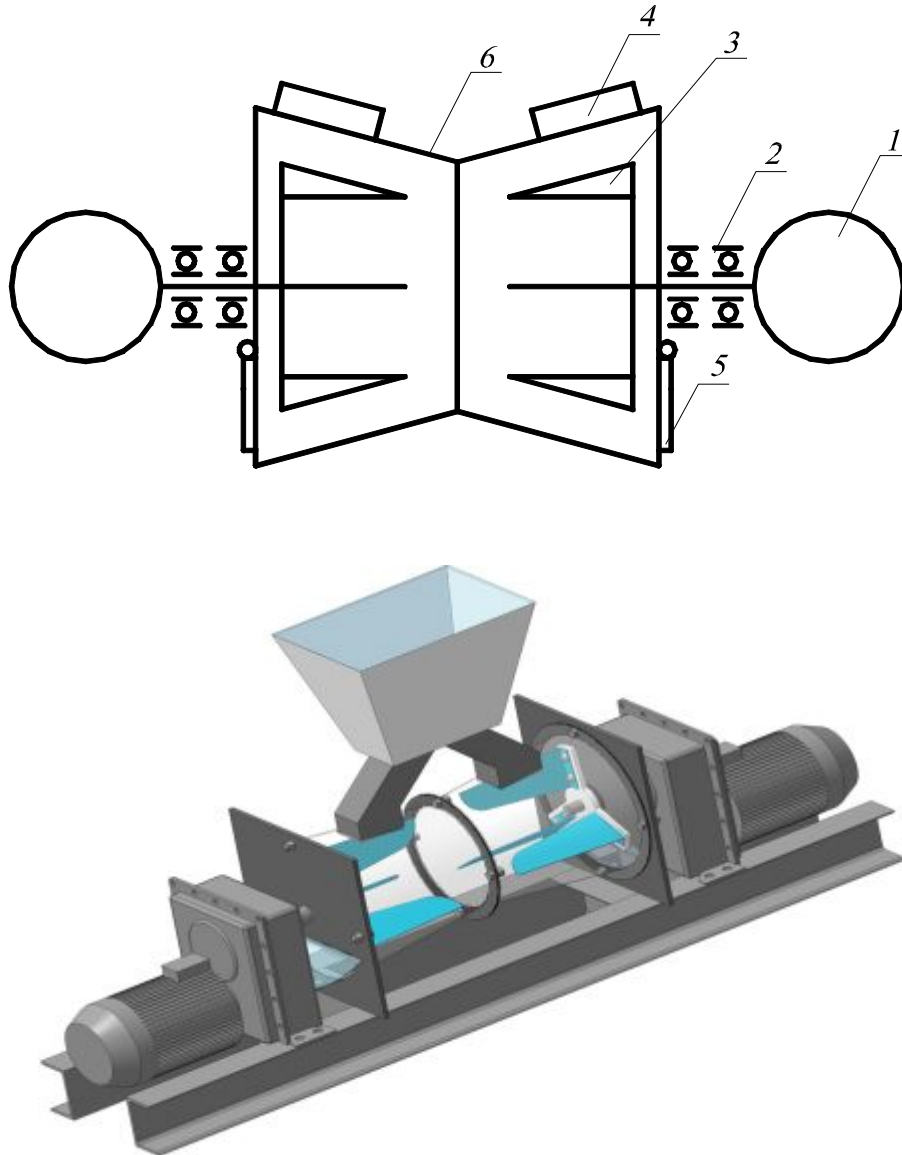
Рис. 3. Кинематическая схема противоточно-турбулентного смесителя 1 – мотор-редуктор; 2 – подшипниковые опоры; 3 – ротор; 4 – загрузочный патрубок; 5 – заслонка разгрузочного отверстия; 6 – корпус
