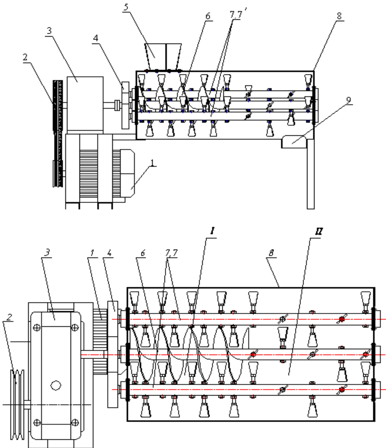
Рис. 1. Конструктивная схема трехвального бетоносмесителя:
