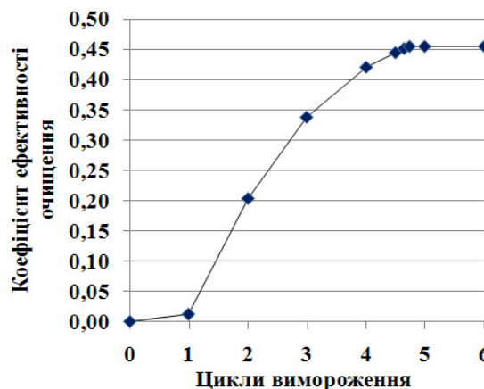
Рис. 4 – Розраховані залежності коефіцієнту ефективності очищення води від кількості циклів її заморожування
