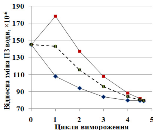
Рис. 2 – Залежність відносної зміни ПЗ водопровідної води від кількості циклів її заморожування: для вимороженої води (сині ромби), не замерзлої води (червоні квадрати) та еквідистантних точок (чорні квадрати)
