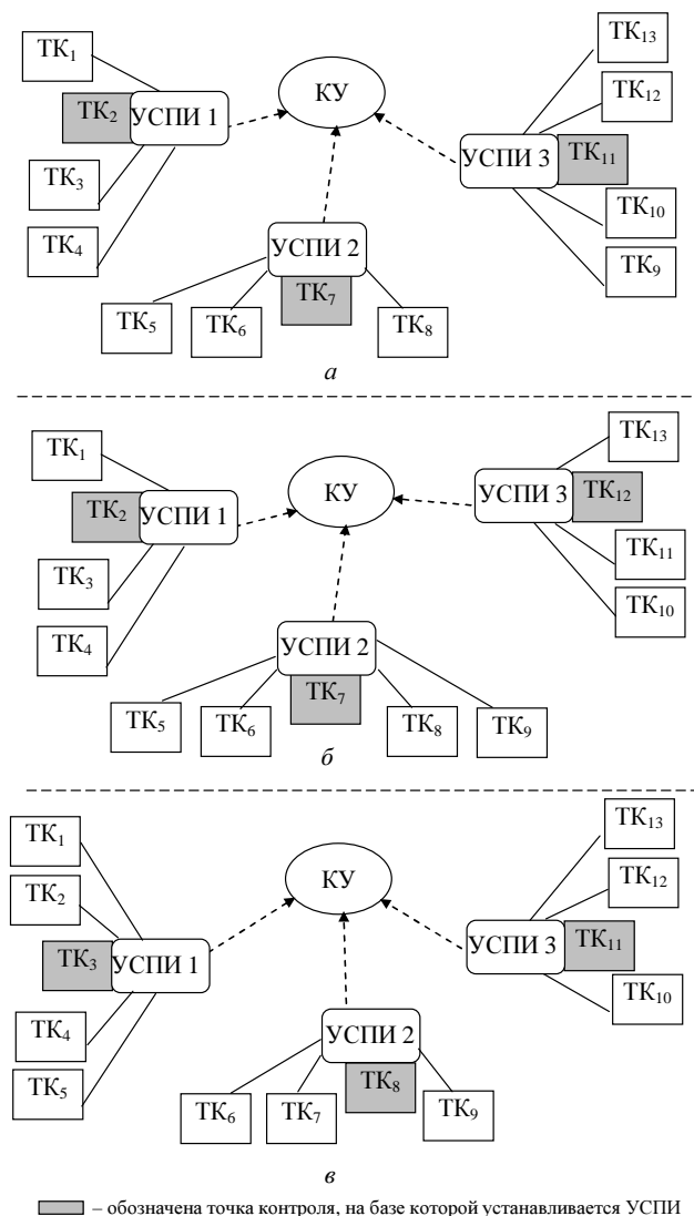
Рис. 3 – Графическое представление структурно-топологической организации СМРГ на участке низкого давления: а – 1-й вариант; б – 2-й вариант; е – 3-й вариант.
