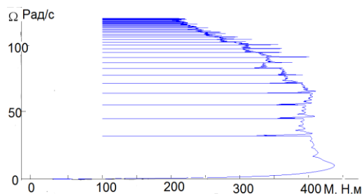
Рис. 4 – Зависимость угловой скорости от среднего значения момента в процессе регулируемого пуска
