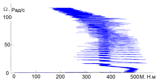
Рис. 5 – Зависимость угловой скорости от мгновенного значения момента при регулируемом пуске
