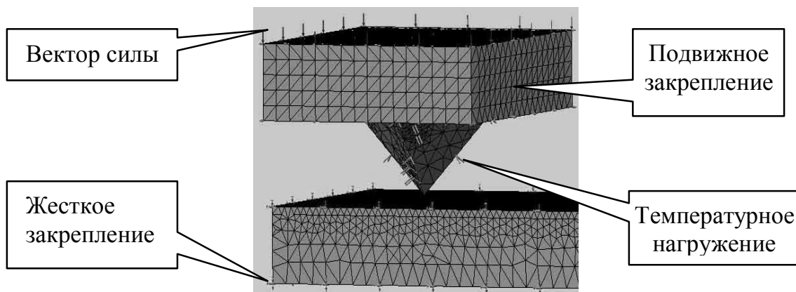
Рисунок 1 – Задание параметров нагружения модели системы «связка–зерно–металлофаза–обработываемый материал»
