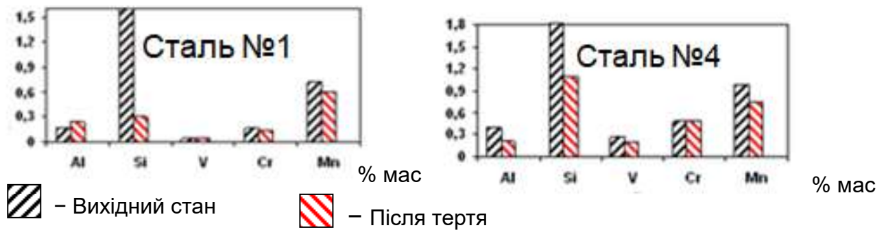
Рис. 3. Вміст елементів на поверхні зразків до і після тертя
