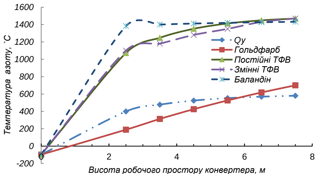
Рис. 1 – Зміна температури газоподібного азоту за висотою робочого простору конвертера
