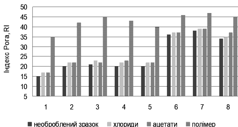
Рисунок. 1. Вплив профілактичних реагентів (2,5 % добавки) на спікливу здатність за методом Рога, (1-8 № проби)
