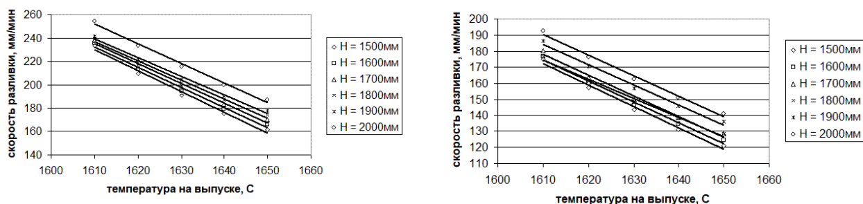
Рис.1. Зависимость скорости разливки стали от температуры металла для девяти и двенадцати дюймовых изложниц (обозначения у линий высота налива изложницы)
