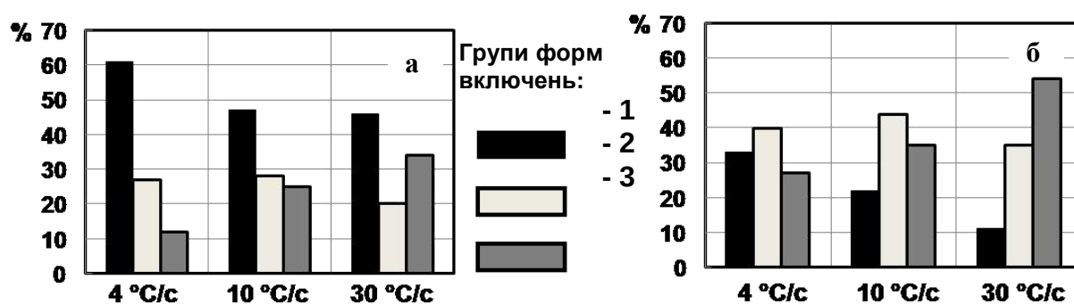
Рис. 2 – Зміна кількості включень з різними формами залежно від швидкості охолодження і індукції магнітного поля: а – В = 0 Тл, б – В ~ 0,1 Тл.
