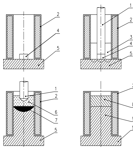
Рис. 1 - Схема відновлення деталей.
