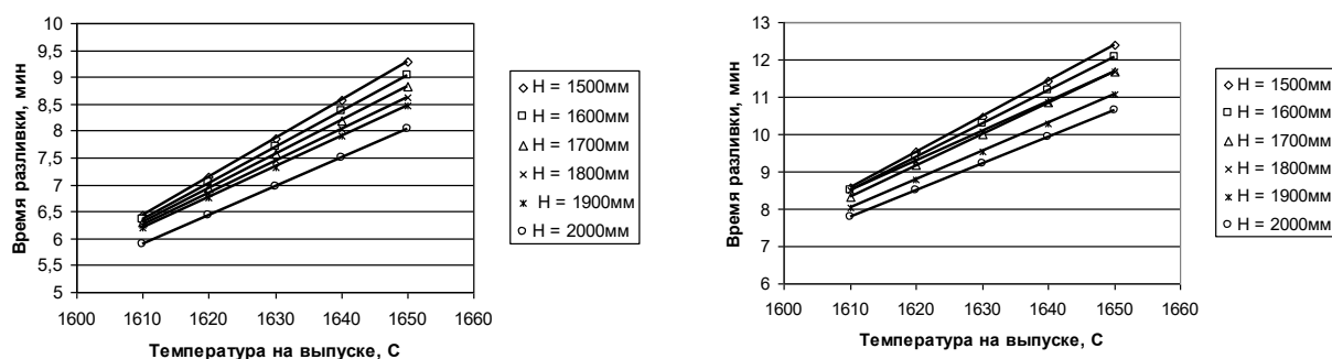
Рис.2. Зависимость времени разливки от температуры металла на выпуске для девяти и дюймовых изложниц
