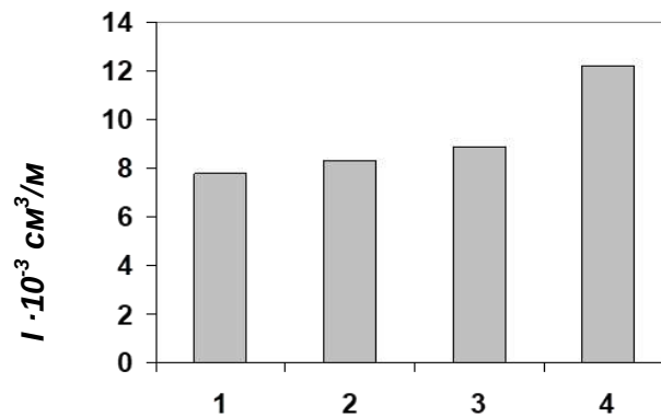
Рис. 2 - Порівняння величини зносу при V=0,2 м/с P=6,4 кг/см 2 деяких композиційних матеріалів:
