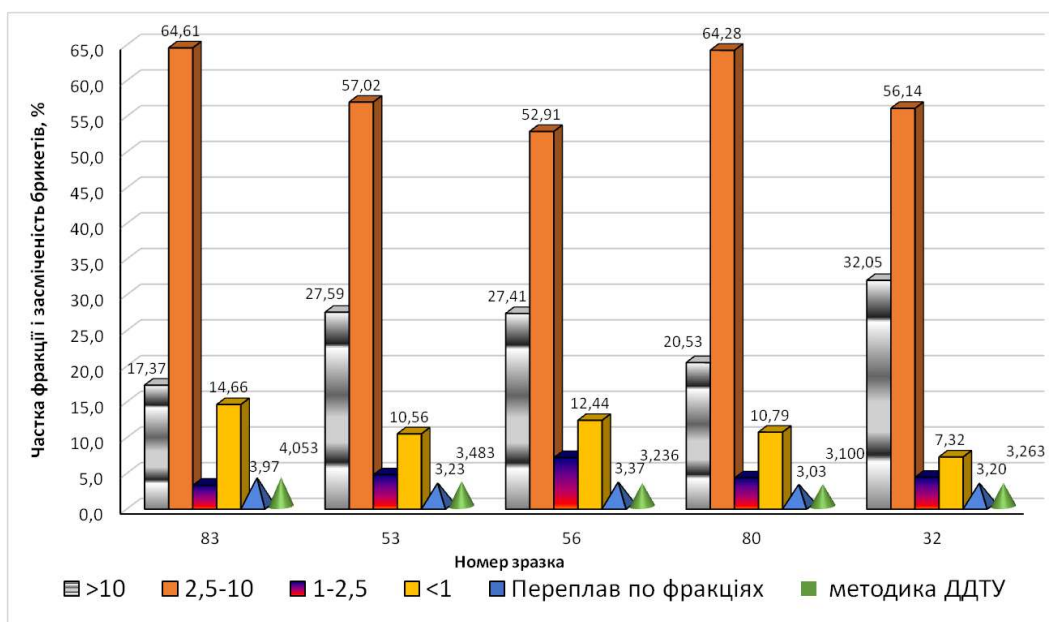
Рис. 1 - Фракційний склад дослідних зразків брикетів та відсоток їх засміченості усіма видами домішок та включень, визначений за компіляційною методикою та МВКЗ-2018 (ДДТУ)
