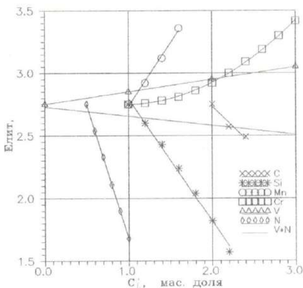
Рис. 1. Вплив елементів на ливарну усадку конструкційної сталі. Температура заливки - 1550 °С. Вміст C і V становить 0,1; N-0,01; N-V-0,001 частку значень наведених на осі абсцис.
