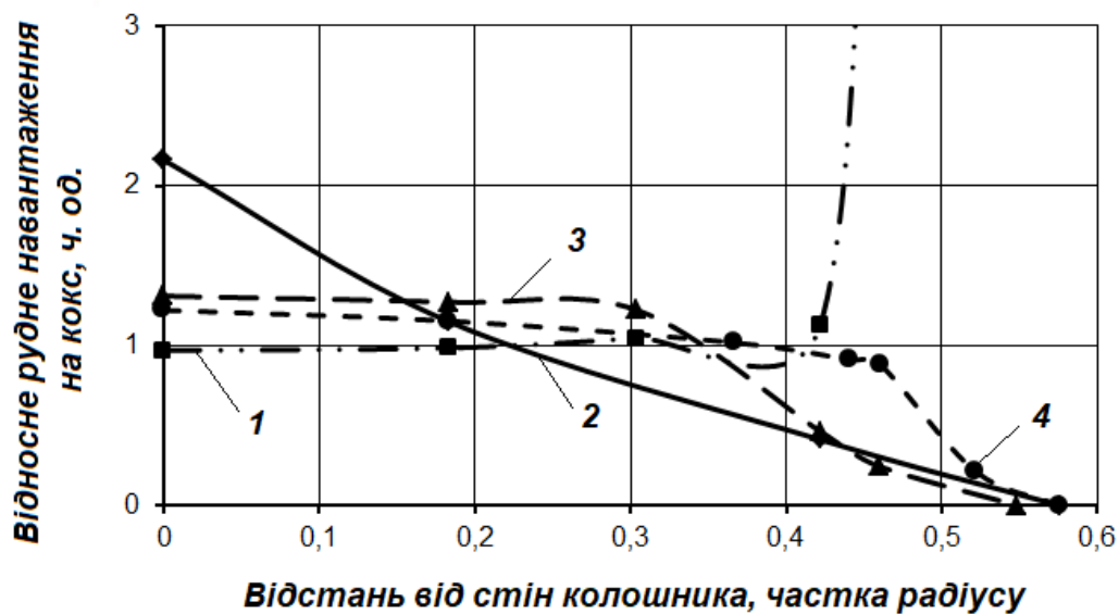
Рис. 1 Результати моделювання зміни РРН при завантаженні доменної печі по циклах: 1 – 4A \downarrow 4K \downarrow ; 2 – 3A \downarrow 4K \downarrow ; 3 – K 2A \downarrow 2A 3K \downarrow ; 4 – 2K A \downarrow 3A 2K \downarrow
