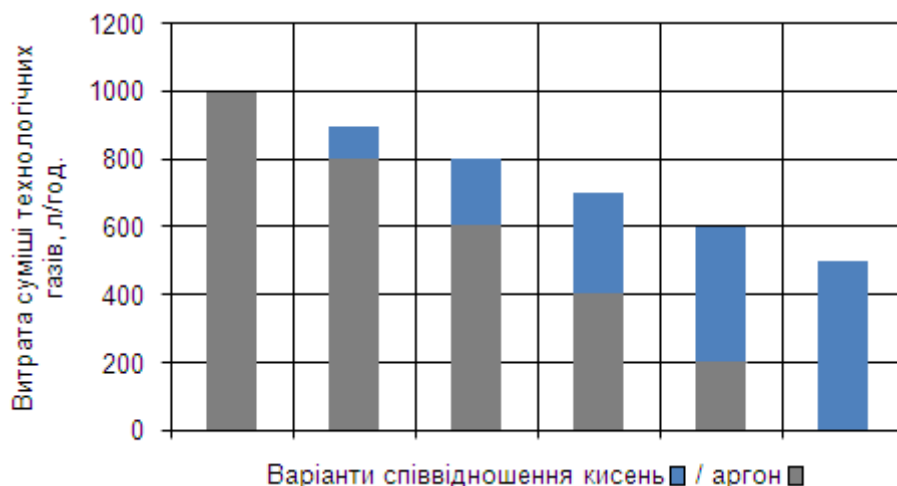
Рис. 1 – Витрати суміші технологічних газів (аргон-кисень) для рафінування металу у ковші
