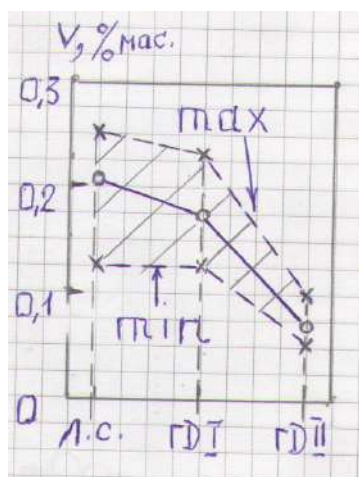
Рис. 2. Максимальний, мінімальний і усереднений вміст ванадію у мікрооб'ємах сталі в литому стані і після гарячої деформації по режимах 1 і 2.
