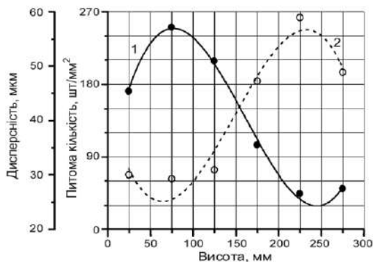
Рис. 2 – Зміна трибоструктури ЛКМ системи [Al – FeCr] по висоті виливка: 1 – дисперсність АФ; 2 – питома кількість включень АФ
