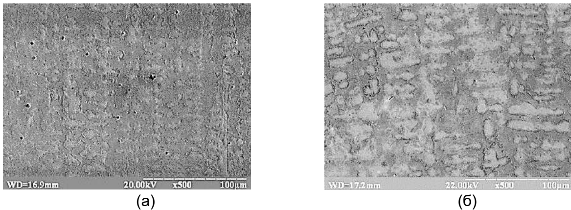
Рис. 2 – Мікроструктура зразків сплавів, що кристалізувались при швидкості охолодження розплаву 250 °C/c Fe-20Mn-12Al-1C (а) та Fe-20Mn-12Al-1C-0,1La (б)
