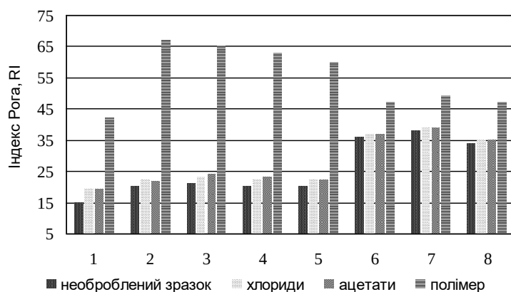
Рисунок 2. Вплив профілактичних реагентів (5 % добавки) на спікливу здатність за методом Рога (1-8 № проби)
