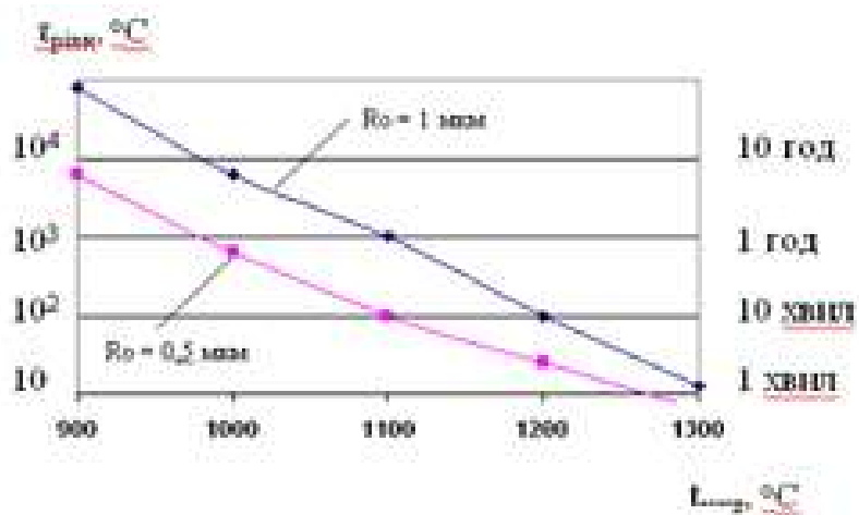
Рис. 3. Час досягнення рівноважності у системі [V],[N] \rightarrow VN в залежності від температури і вихідного розміру частинок VN ( R_0 )
