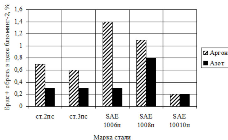
Рис. 2. Сравнительный анализ качества металла, выплавленного с применением аргона и азота
