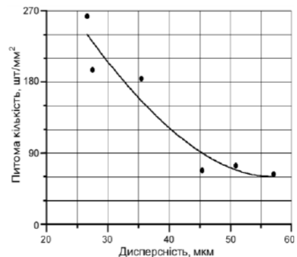
Рис. 3 – Вплив середньої дисперсності часток армуючої фази на питому кількість їх включень в об’ємі литих зразків
