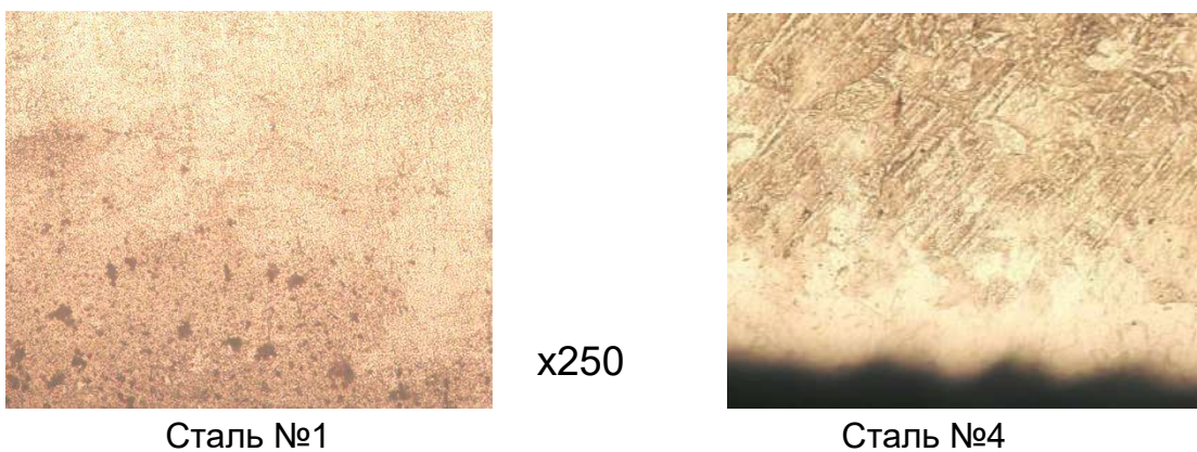
Рис. 4. Мікроструктура зони руйнування зразків при випробуванні на втомну витривалість
