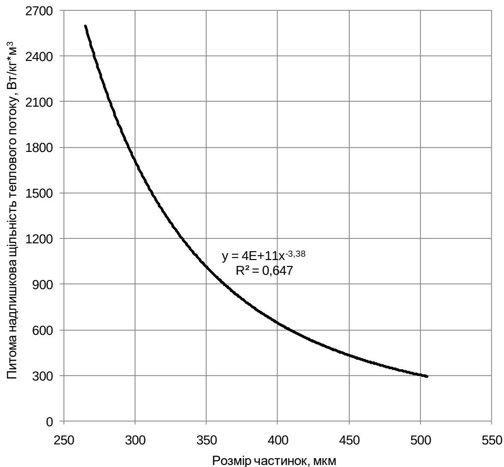
Рис.1 – Вплив розміру твердих частинок на величину питомої надлишкової щільності теплового потоку випромінюванням
