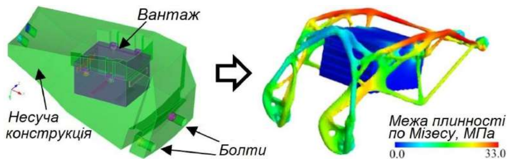
Рис. 1. Приклад проєктування легковагої конструкції кронштейну.
