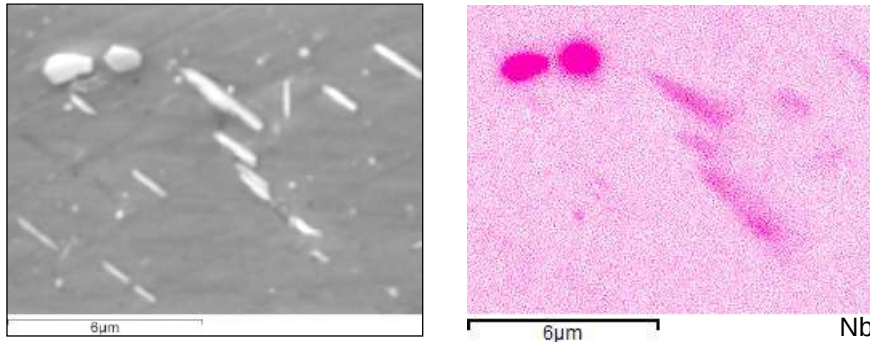
Рис. 1 Результати рентгеноспектрального мікроаналізу у місцях розташування \delta -фази у режимі картирування. Більшому вмісту елементу відповідає більш інтенсивне забарвлення
