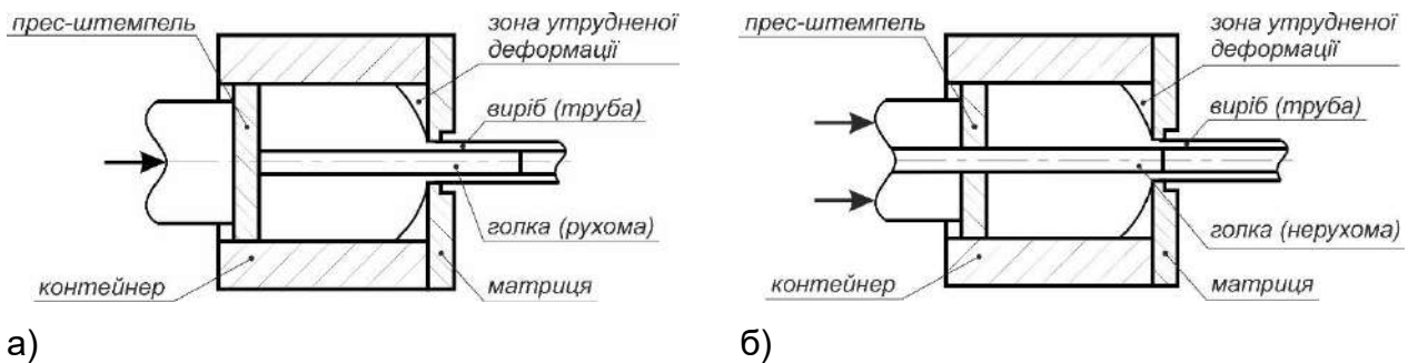
Рисунок 1 – Схеми прямого пресування труб з рухомою (а) та нерухомою (б) голкою
