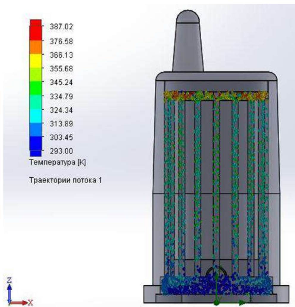
Рис. 2 – Розподіл середньої температури повітря в каналах стержня
