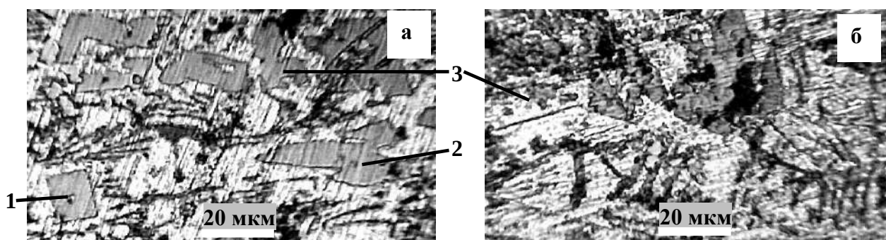
Рис. 1 – Форми включень у сплаві Al - 3,7Cu -13 % РЗМ: а – В = 0 Тл, б – В ~ 0,1 Тл.
