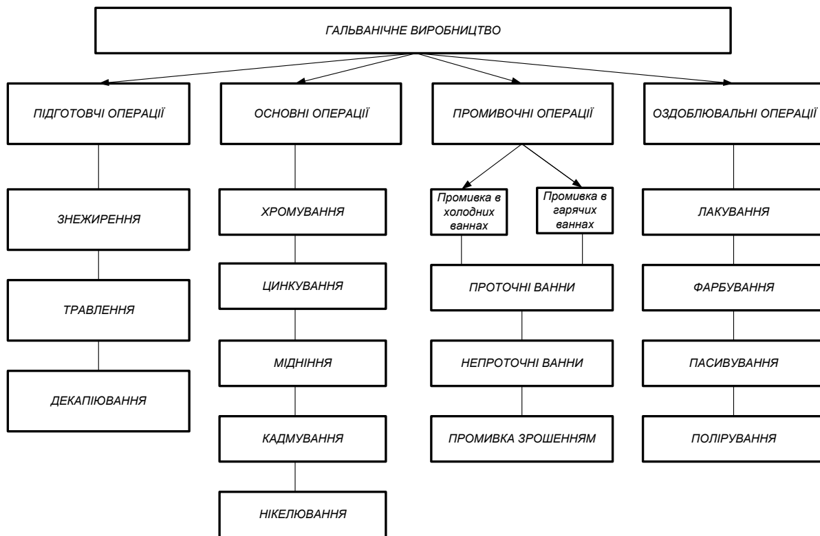
Рис.1 – Технологічні операції при нанесенні гальванічного покриття
