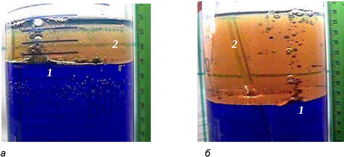
Рис. 1 - Вигляд формування «проривної» металеві зони (тунелю) 1 на границі «метал-шлак» 2 у шлаковому шарі товщиною 30 (а) та 70 мм (б)
