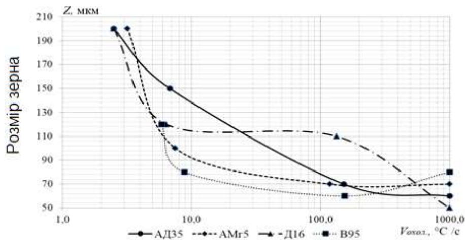
Рис. 1 - Вплив швидкості охолодження на розмір зерна алюмінієвих сплавів
