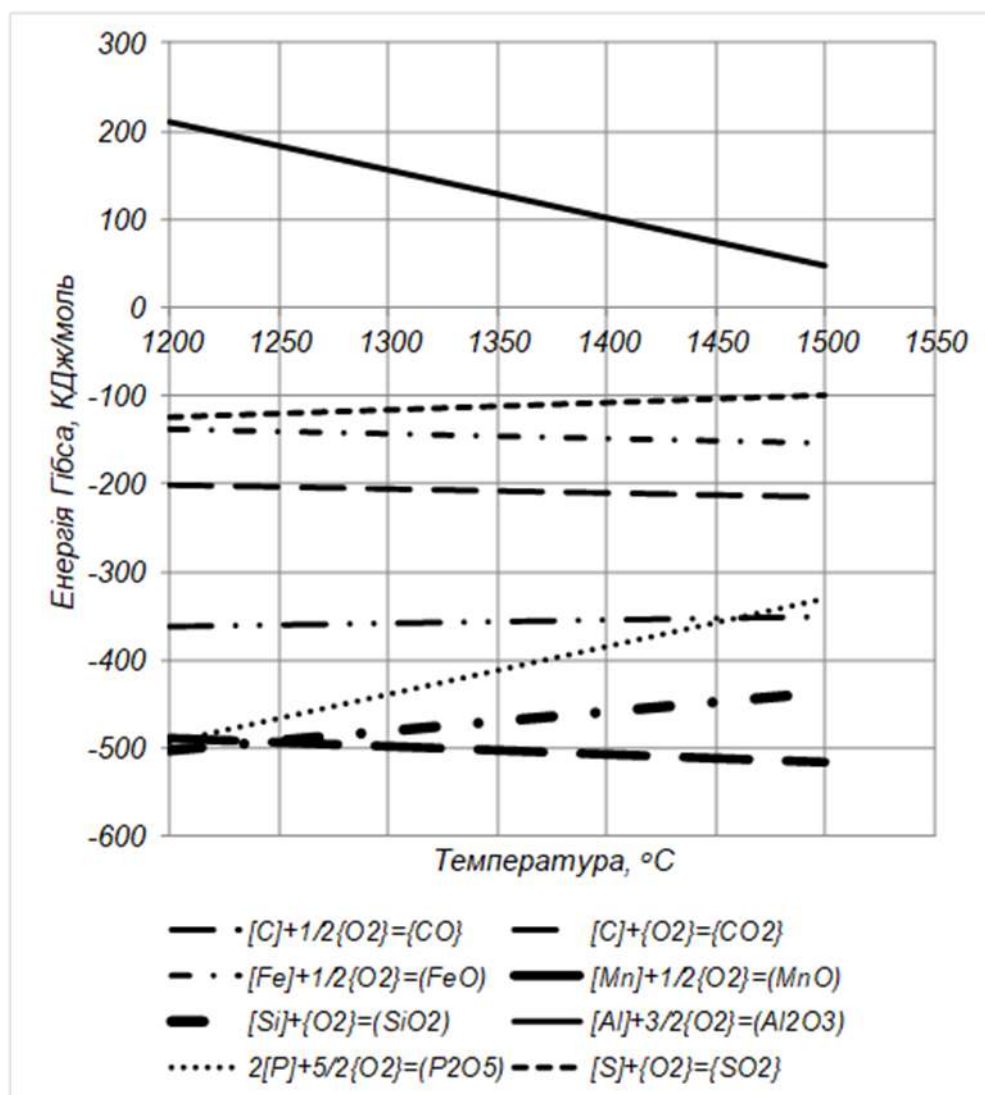
Рис. 1 – Графічна залежність енергії Гібса від температури для процесів взаємодії компонентів рідкого чавуна з газоподібним киснем при одночасній десульфурзації та десиліконізації
