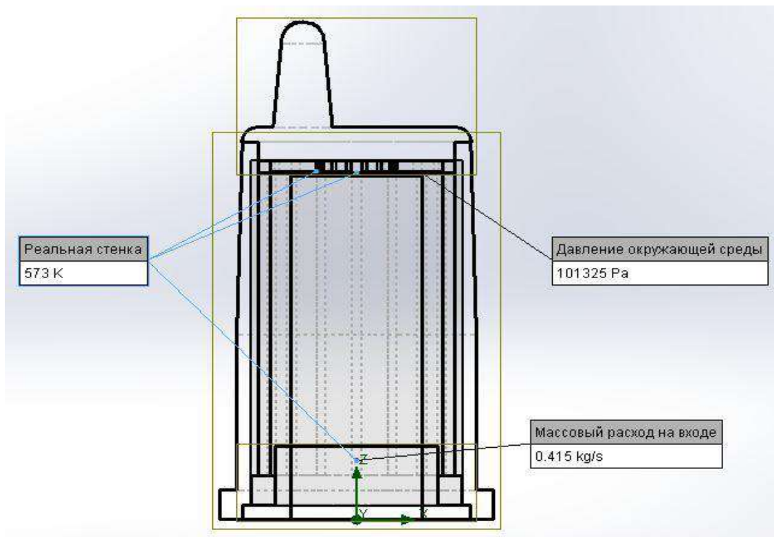
Рис. 1 – Граничні умови розрахункової області на вході і виході
