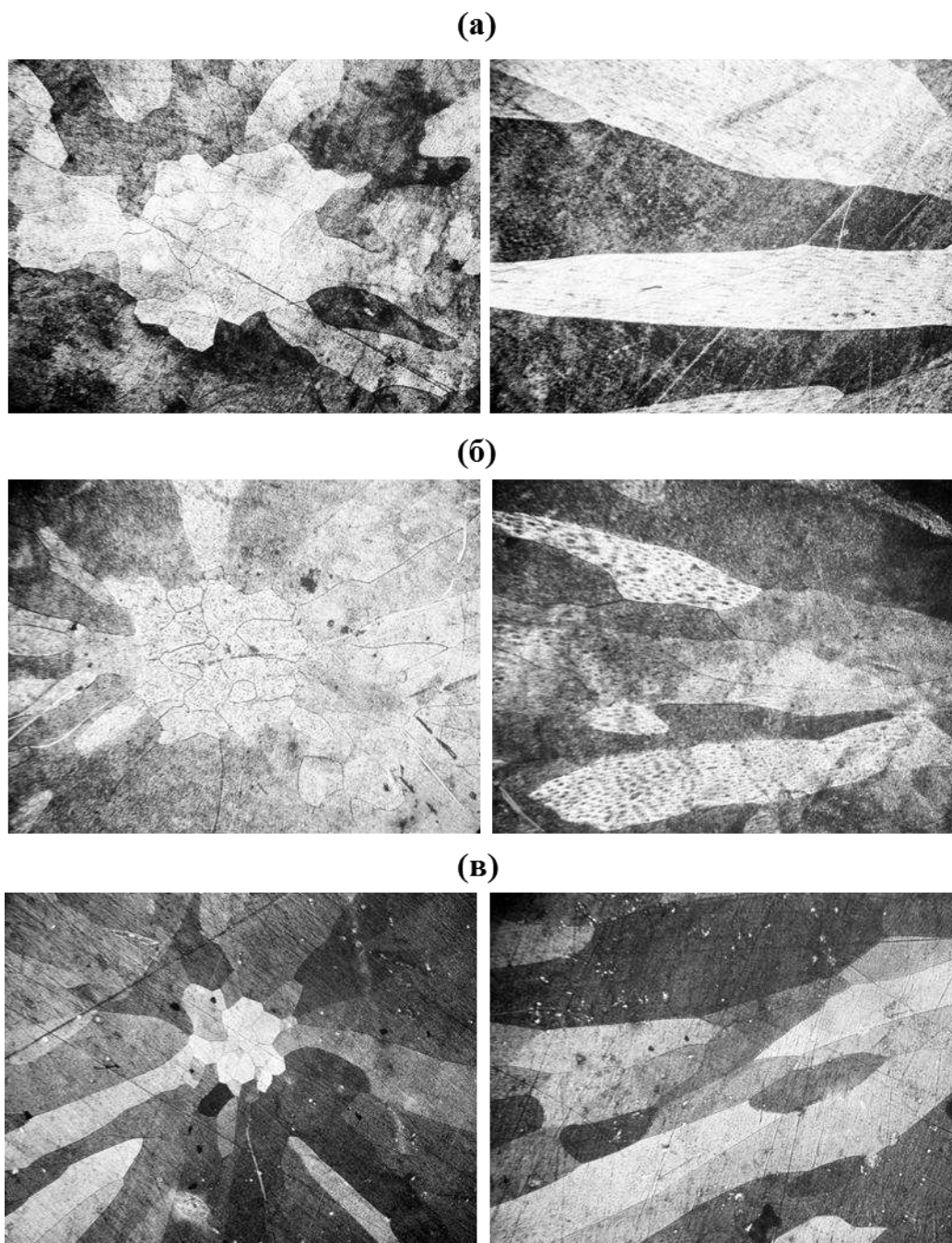
Рис. 1. Мікроструктура міді після витяжки: а) шаг 3,3 мм, б) 8,2 мм, в) 16,8 мм, x100
