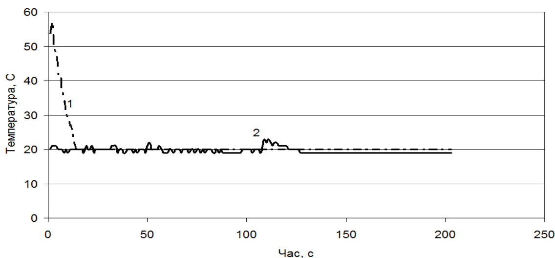
Рис.1 -- Охолодження ПФ в потоці води 1-температура стінки ПФ; 2-температура вод
