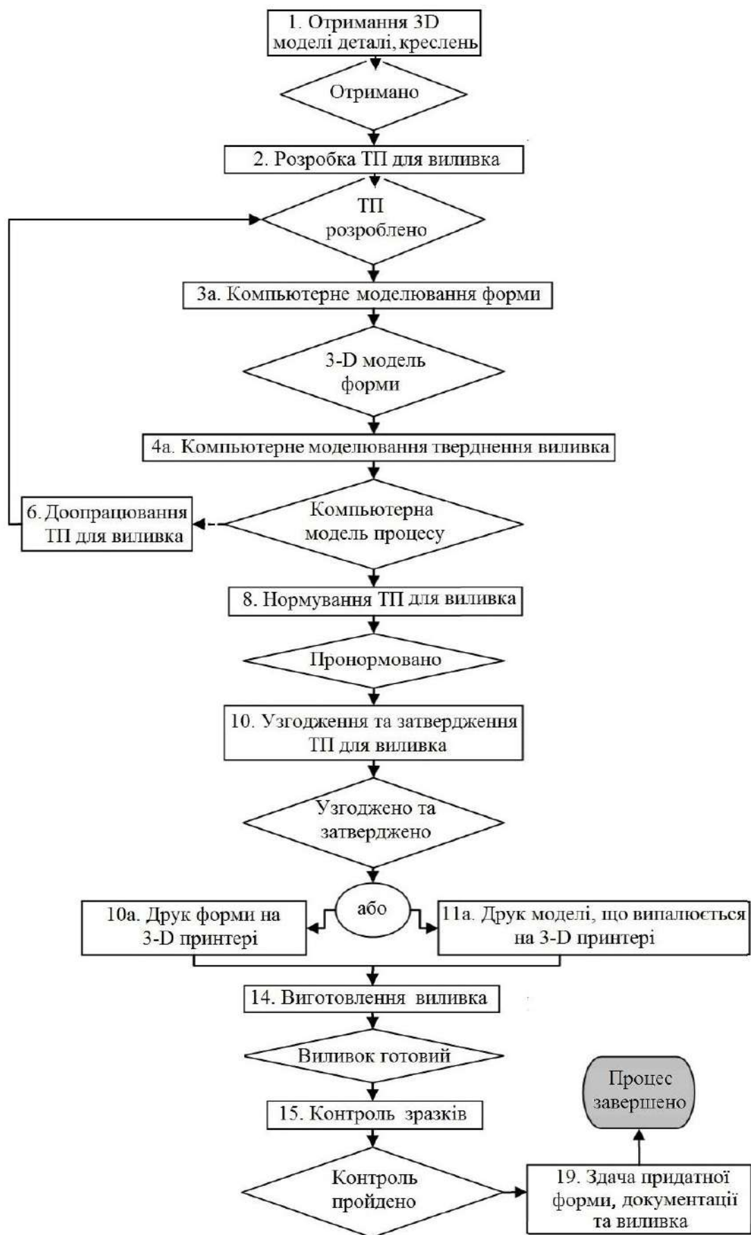
Рис. 3. Схема КТПВ із застосуванням 3D цифрових технологій.
