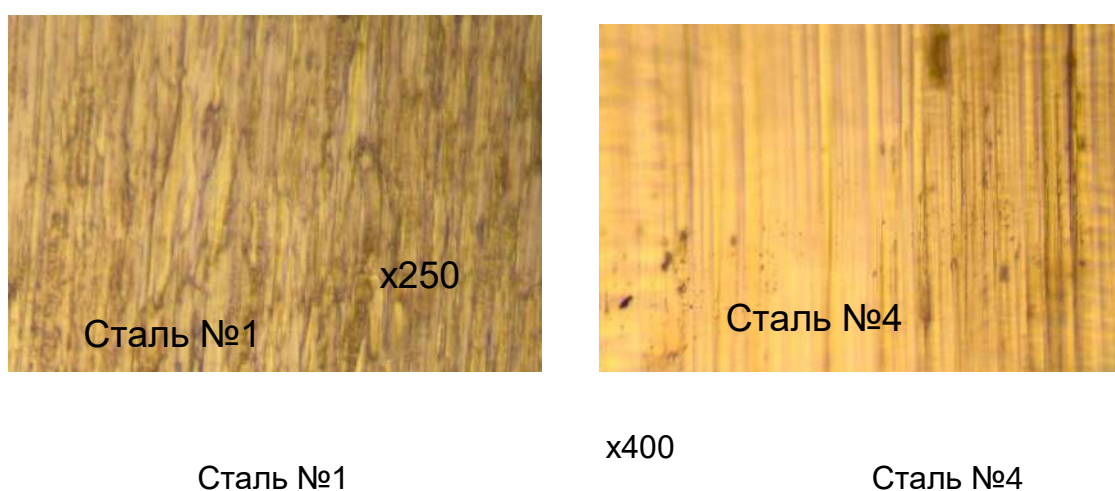
Рис. 4. Структура поверхні після зношування стандартної сталі №1 і №4 з комплексним зміцненням
