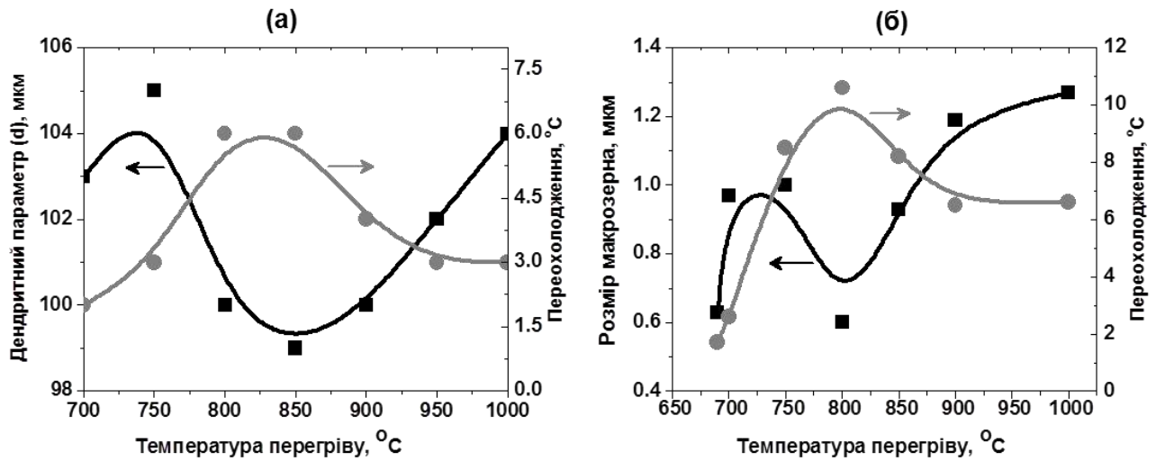
Рис. 1 – Вплив температури перегріву та переохолодження на дендритний параметр (а) і розмір макрозерна (б) в зразках з високоміцного алюмінієвого сплаву В96ц
