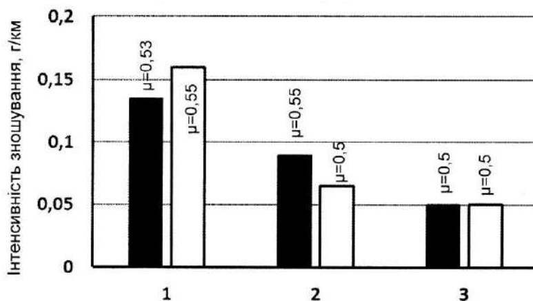
Рис. 2 — Інтенсивність зношування стандартної сталі 95Х18 (1) і дослідних литих сталей 120Х15Г (2) і 120Х15Б (3) в умовах граничного тертя до (■) і після плазової-детонаційної обробки (□).
