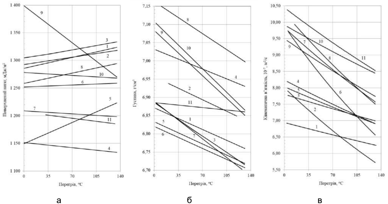
Рис. 1 - Політерми поверхневого натягу (а), густини (б) і кінематичної в'язкості (в) досліджених розплавів низько- і середньолегованих конструкційних сталей.
