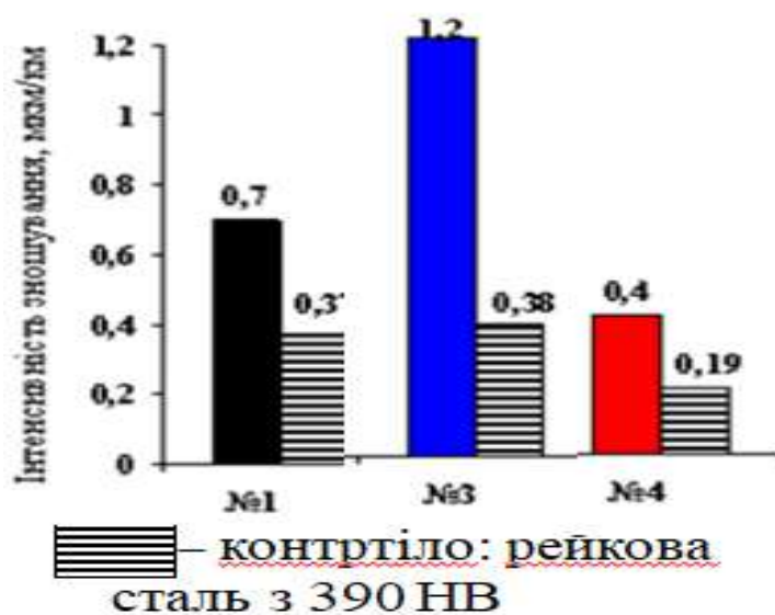
Рис. 1 Інтенсивність зношування дослідних сталей в умовах сухого тертя коченням ( V=2,4 м/с, P=140 МПа, l=6,8 км)
