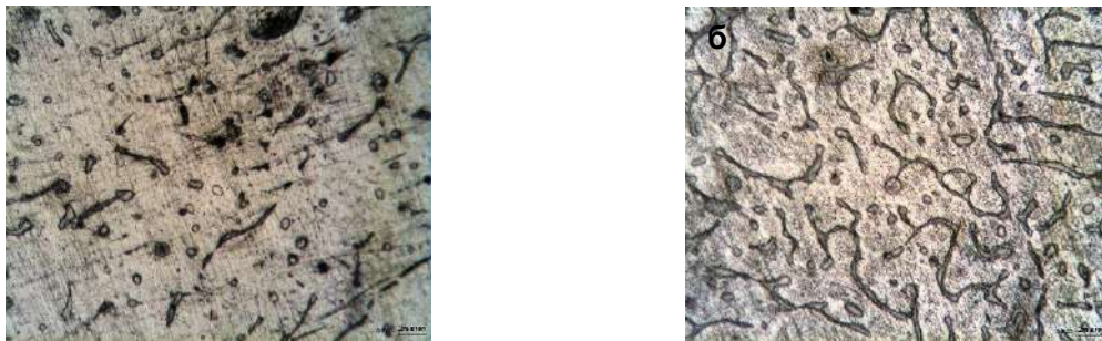
Рис. 1 – Мікроструктура сплавів алюміній-олово (а - зразок 1; б - зразок 2) x500.
