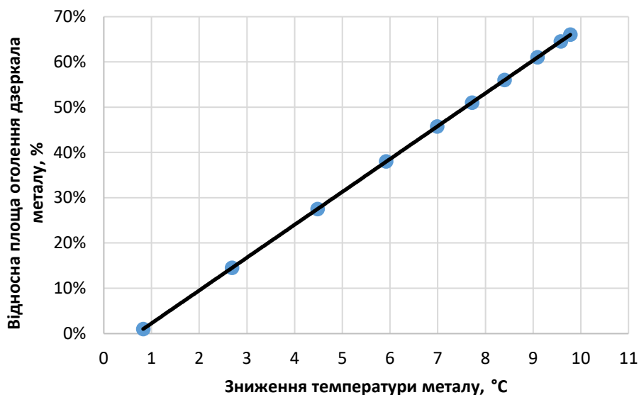
Рис. 2 – Залежність зниження температури сталі від витрат газу за весь період продувки на установці «ківш-піч»
