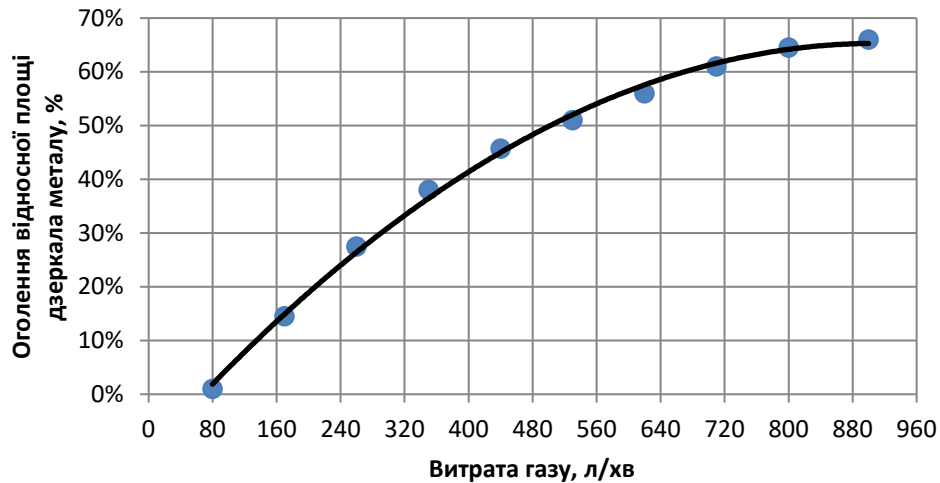
Рис. 1 – Залежність оголення відносної площі дзеркала металу від витрат газу
