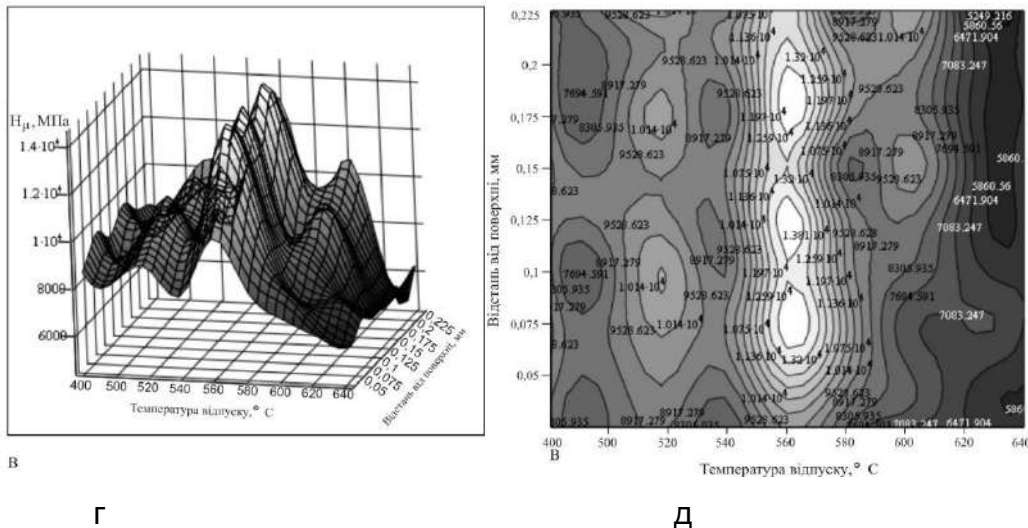
Рис. 1 – Залежність (а, в) і розподіл (б, д) мікротвердості по глибині дифузійного шару дослідних зразків від температури відпуску; а, б - сплав 20P18, в, д - сплав 20P6M5
