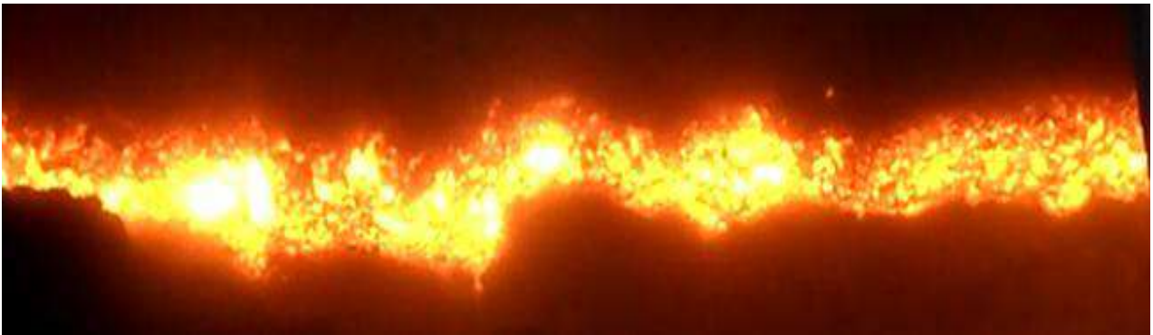
Рисунок 3 – Фото високотемпературної зони по ширині палети при формуванні шару шихти з використанням розподільника шихти
