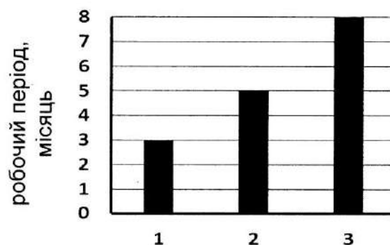
.Рис. 1 – Результати випробувань ущільнювальних кілець, виготовлених з різних матеріалів на насосах НК 200/370 в промислових умовах: 1 - сталь 40X, 2 - сталь 20 з наплавленням Сормайт, 3 - лита сталь 120X15Г.
