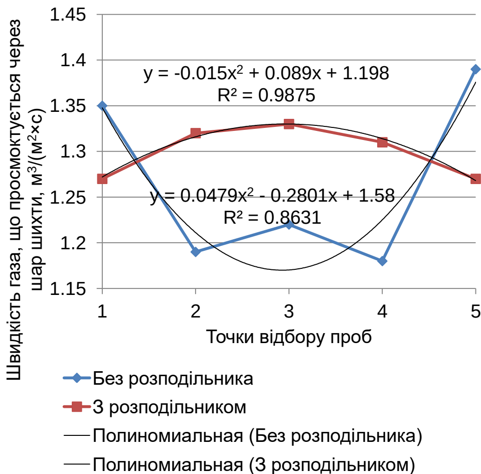
Рисунок 2 – Розподіл газопроникності по ширині палети
