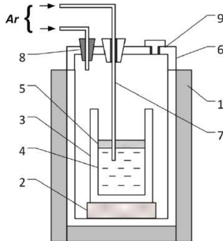
Рисунок – Схема експериментальної установки: 1 – піч Таммана; 2 – керамічна підставка; 3 – алуновий тигель; 4 – метал; 5 – шлак; 6 – кришка; 7 – трубка для інжекції реагентів; 8 – отвір для введення аргону; 9 – отвір для відбору проб
