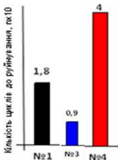
Рис. 2. Втомна витривалість (п циклів до руйнування) дослідних сталей
