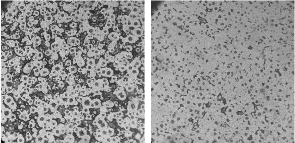
Рис. 1 – Мікроструктура (x100) після травлення чавуну ВЧ 500 і ВЧ400
