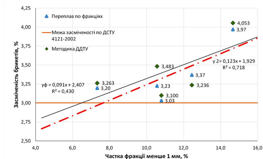
Рис. 2 – Зв'язок частки фракції стружки менше 1 мм з контрольних проб з загальною засміченістю брикетів. Горизонтальна лінія відображає допустиму межу засміченості брикетів сталеної стружки виду №15 (3%)
