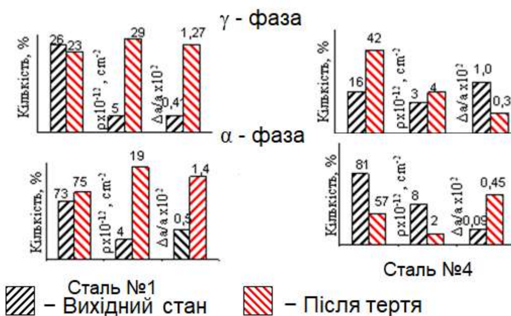
Рис. 3. Фазовий склад і параметри кристалічної ґратки поверхні зношування сталей у вихідному стані і після зношування
