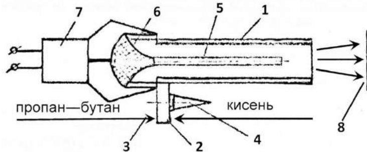
Рис. 1 – Схема пристрою плазово-детонаційної обробки
