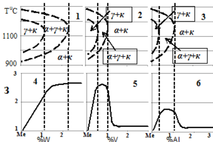
Рис. 1 - Схеми діаграм склад-структура-зносостійкість сталі 120Х15Л, при додатковому роздільному легуванні вольфрамом, ванадієм або алюмінієм. (Функції 4 і 5 побудовані за даними [1, 2]):
