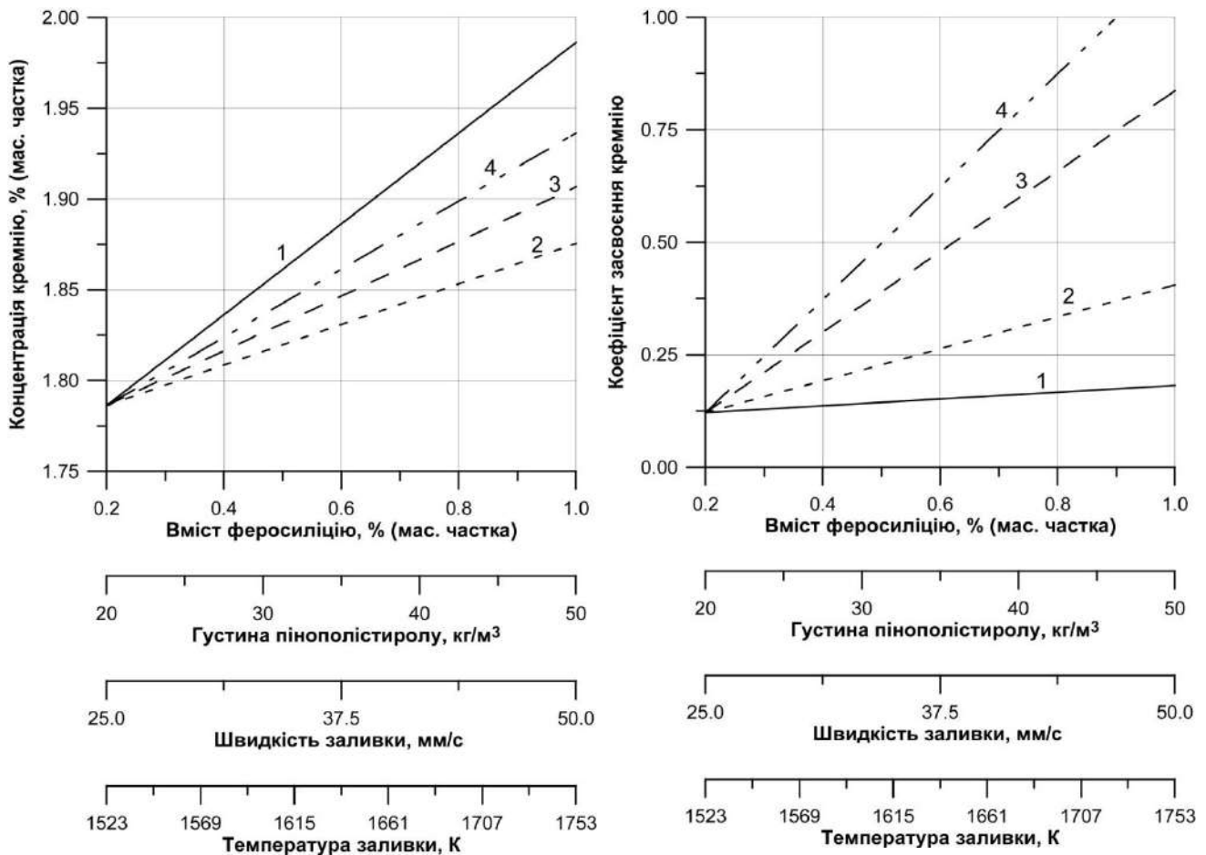
Рис. 1 (лів.) – Залежність концентрації кремнію у чавуні від технологічних параметрів ЛГМ-процесу: 1 – вмісту феросиліцію; 2 – густини пінополістиролу;
