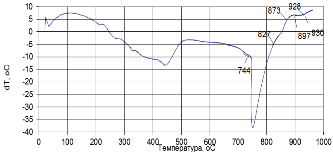
Рисунок 1 - Криві ДТА при нагріві досліджуваної сталі класу С.
