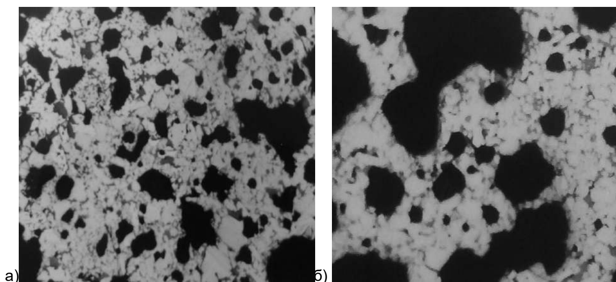
Рис. – Мікрофотографія структур окатишів на основі комплексного флюсу (а) та звичайних (б): світло-сіре – магнетит, біле – гематит, темно-сіре – зв'язка, чорне – пори
