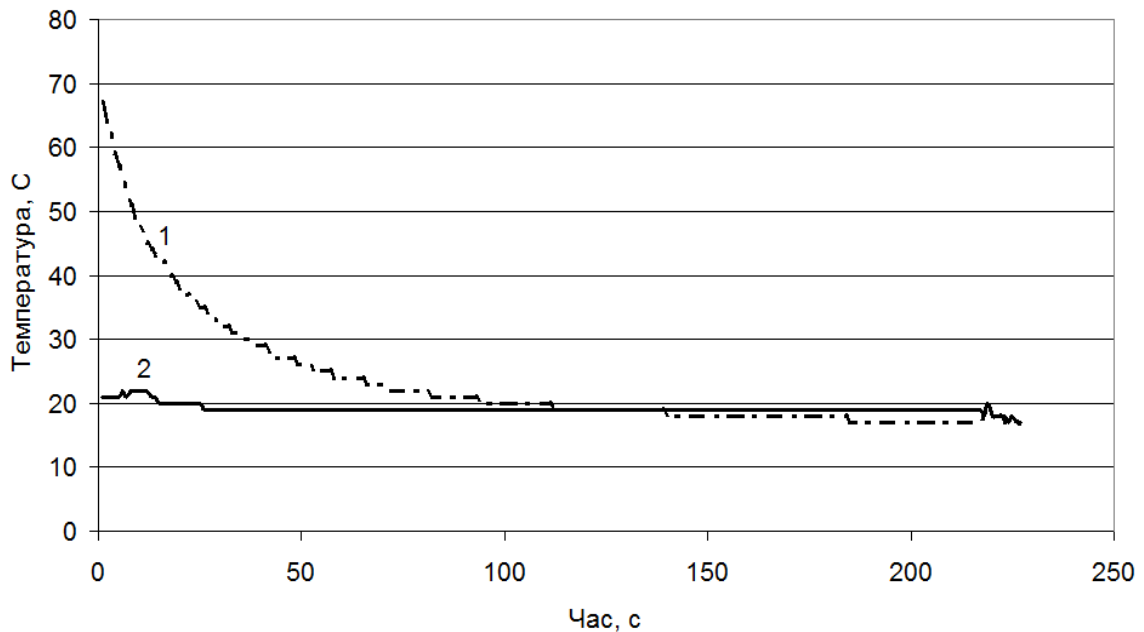
Рис.2 -- Охолодження ПФ в спокійній воді 1-температура стінки ПФ; 2-температура води
