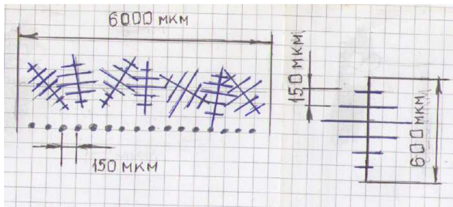
Рис. 1 Схема проведення мікрохімічного аналізу на електронно - растровому мікроскопі SEM-515
