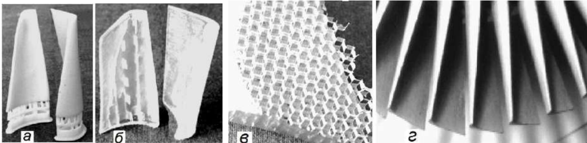
Рис. 3. Приклади друкованих полімерних моделей: а – модель лопаті цільна; б - модель лопаті з двох половин і порожниною після їх склейки; в - стільникова структура розпірок крильчатки; а також г - крильчатка з металевими лопатями, за такими моделями.
