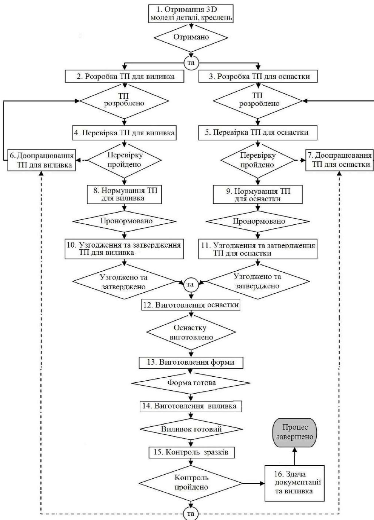
Рис. 2. Схема КТПВ без застосування нових цифрових технологій.
