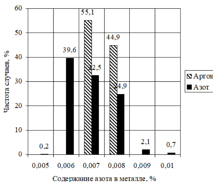
Рис. 1. Частотное распределение содержания азота в стали при использовании аргона и азота в конвертерном цехе
