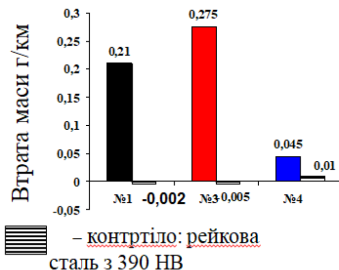
Рис.2. Інтенсивність зношування дослідних сталей при сухому терті ковзанням ( V=1 м/с, P=1 МПа, l=1,2 км)
