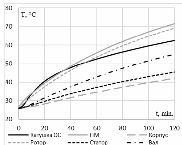
Рис. 10. Нагрев деталей ВДПМ (длительный режим)
