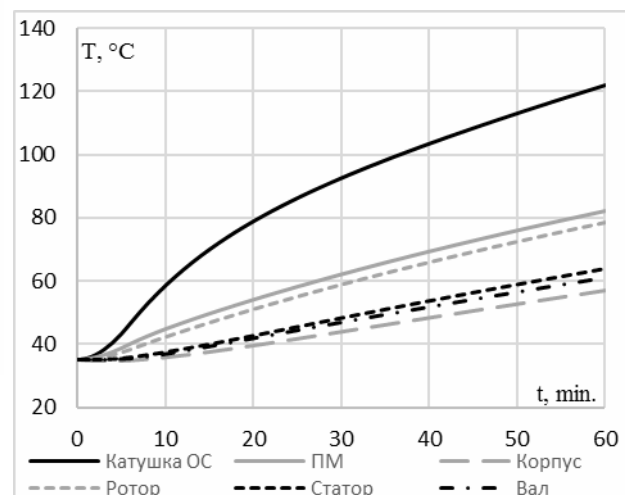
Рис. 9. Нагрев деталей ВДПМ (часовой режим)
