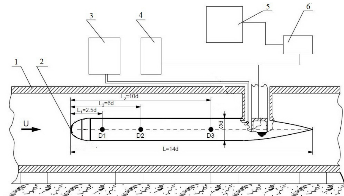
Рис. 1 – Розміщення моделі в гідродинамічній трубі, де: гідродинамічна труба – 1, модель – 2, система подачі полімерів – 3, системи тензометрії і реєстрації шумів – 4, 5, підсилювач сигналів – 6.
