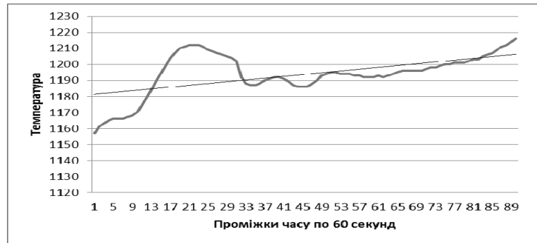
Рис. 7 – експоненціальне усереднення температури у точці Середина на протязі роботи пальників із циклом переключення 30 хвилин
