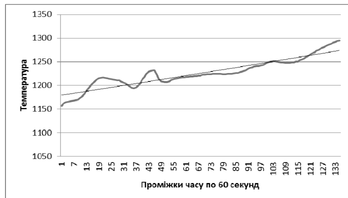
Рис. 9 – експоненціальне усереднення температури у точці Середина на протязі роботи пальників із циклом переключення 45 хвилин
