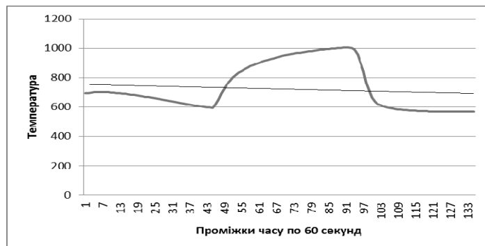
Рис. 8 – експоненціальне усереднення температури у точці Дно 2 на протязі роботи пальників із циклом переключення 45 хвилин
